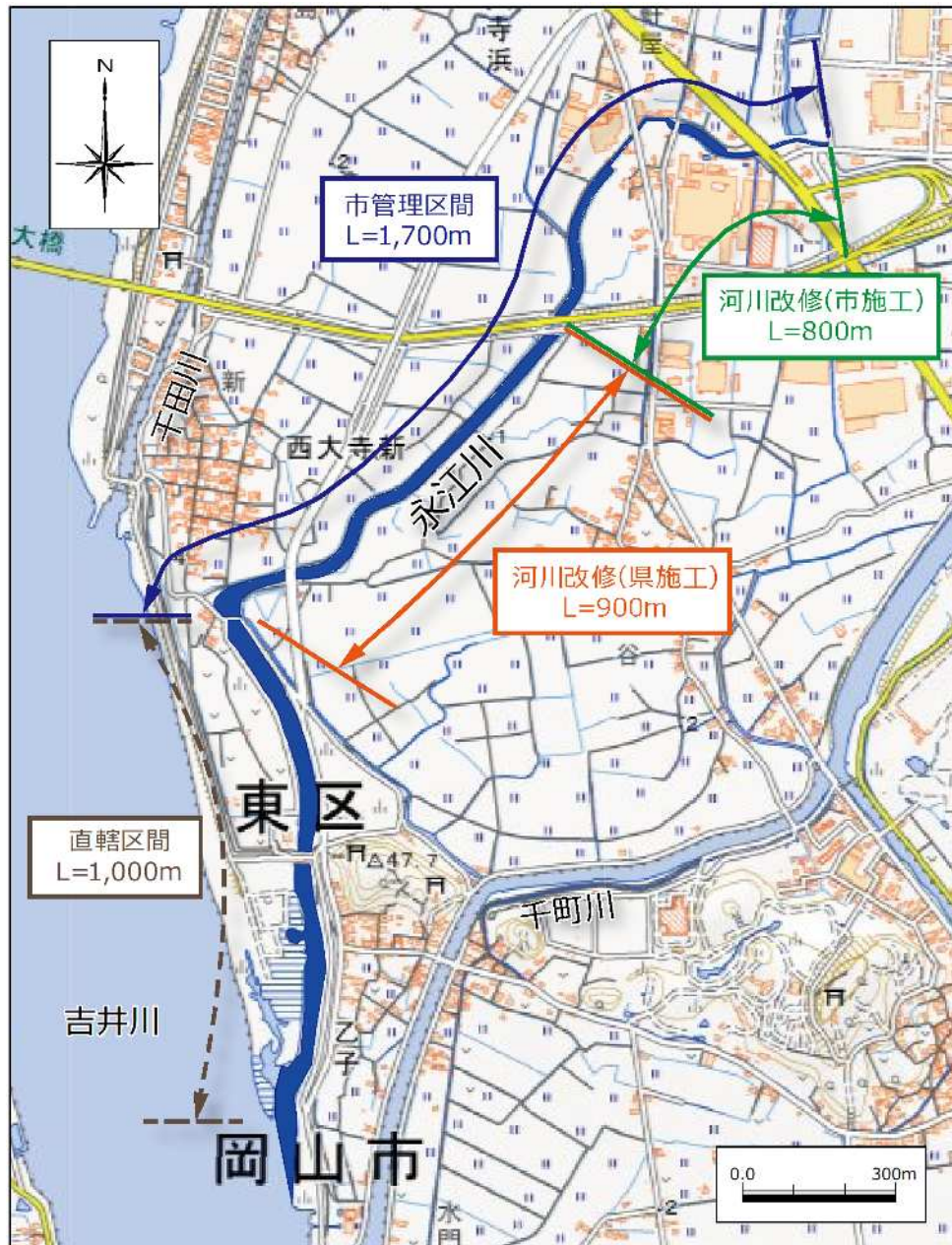
図ー3 永江川関連の河川改修事業位置図
