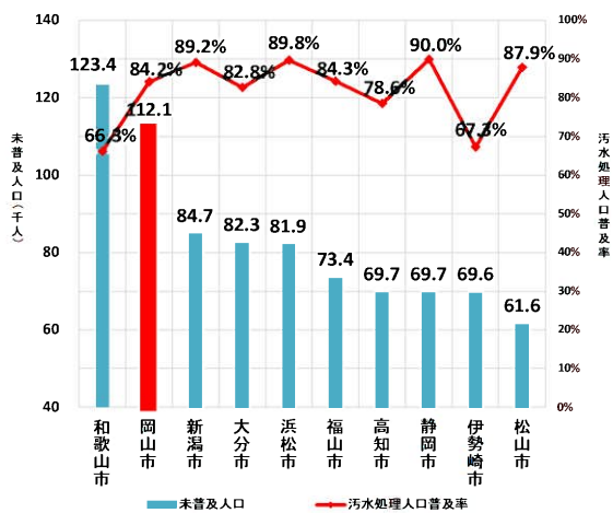
污水处理の未普及人口と污水处理人口普及率の状況
