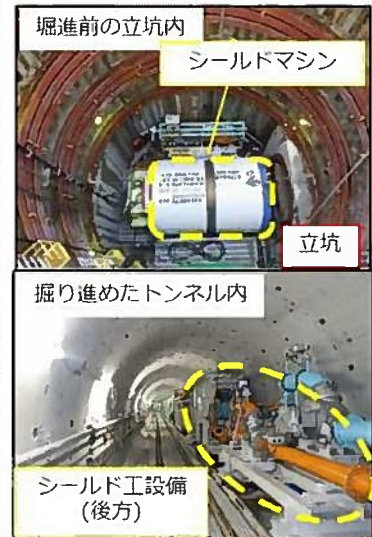
掘進着手（浦安11号雨水幹線）
