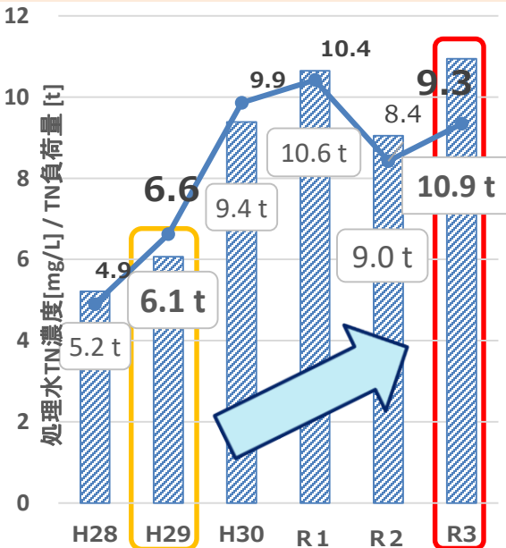
岡東浄化センターにおける冬季（11~3月）の処理水TN/TP平均濃度と負荷量の経年変化
