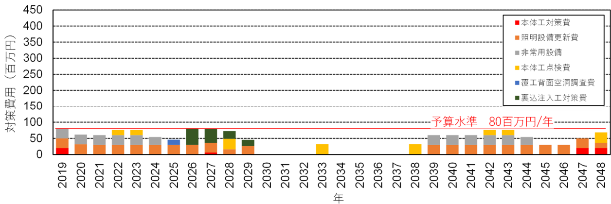
図 2.3 ライフサイクルコスト推定結果（2018 年推計）
