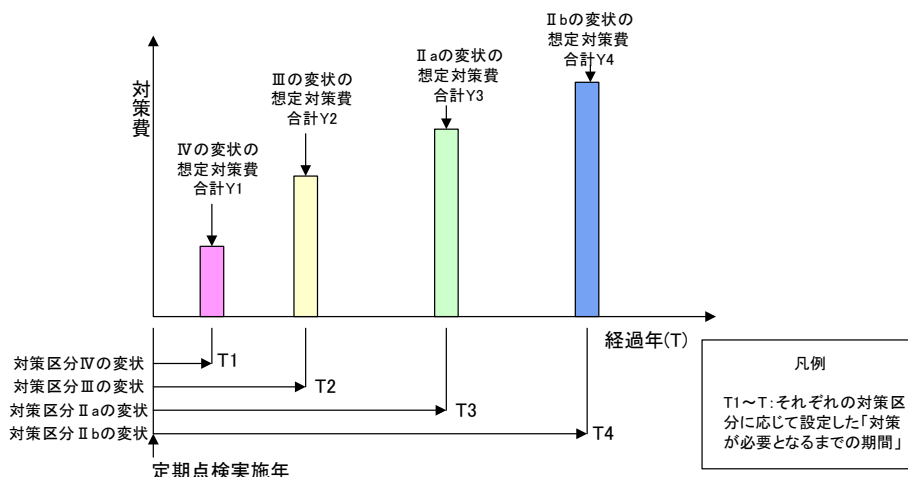
図 2.2 LCC の算出の考え方
