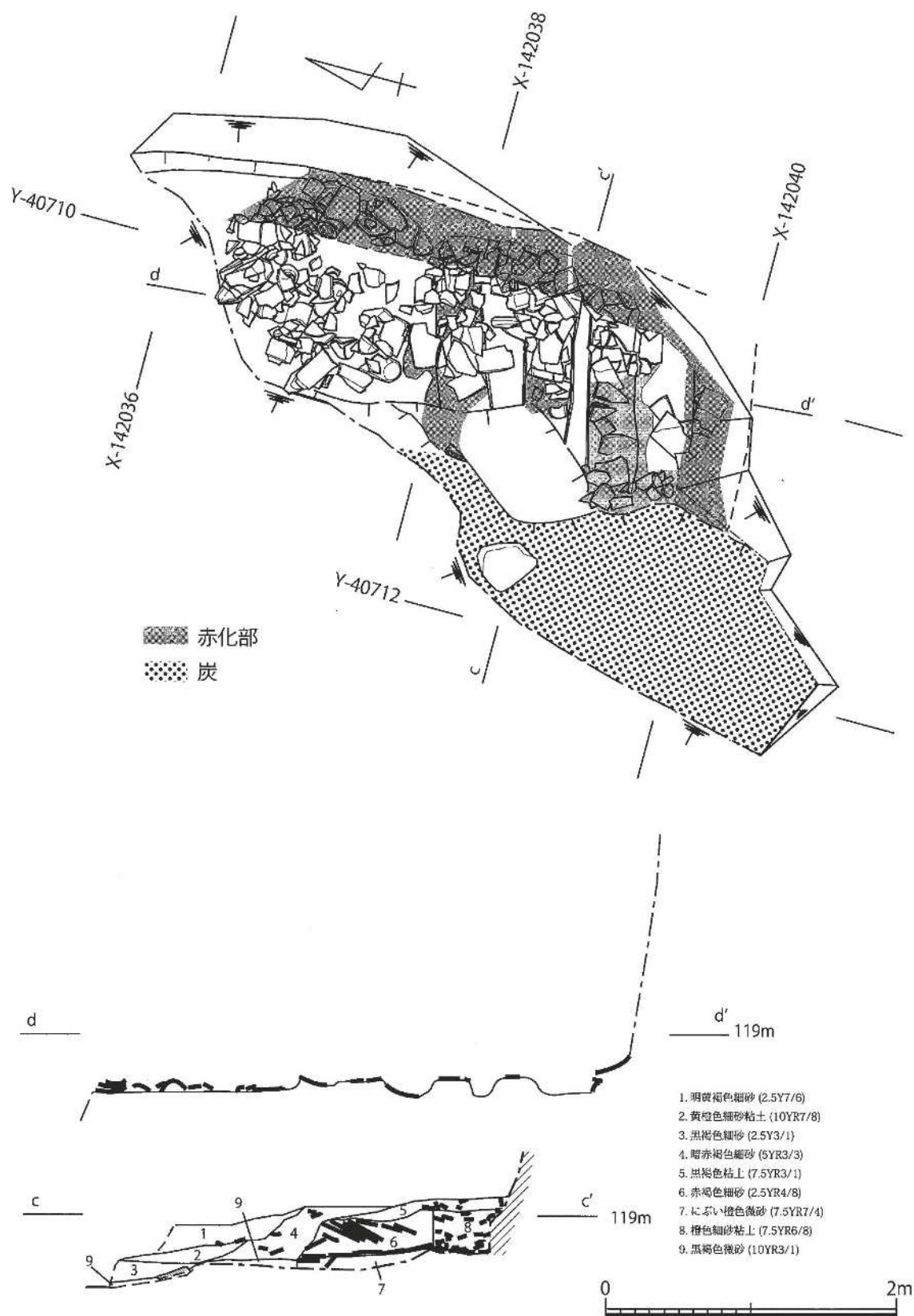
图4 瓦窯平面図・断面図
