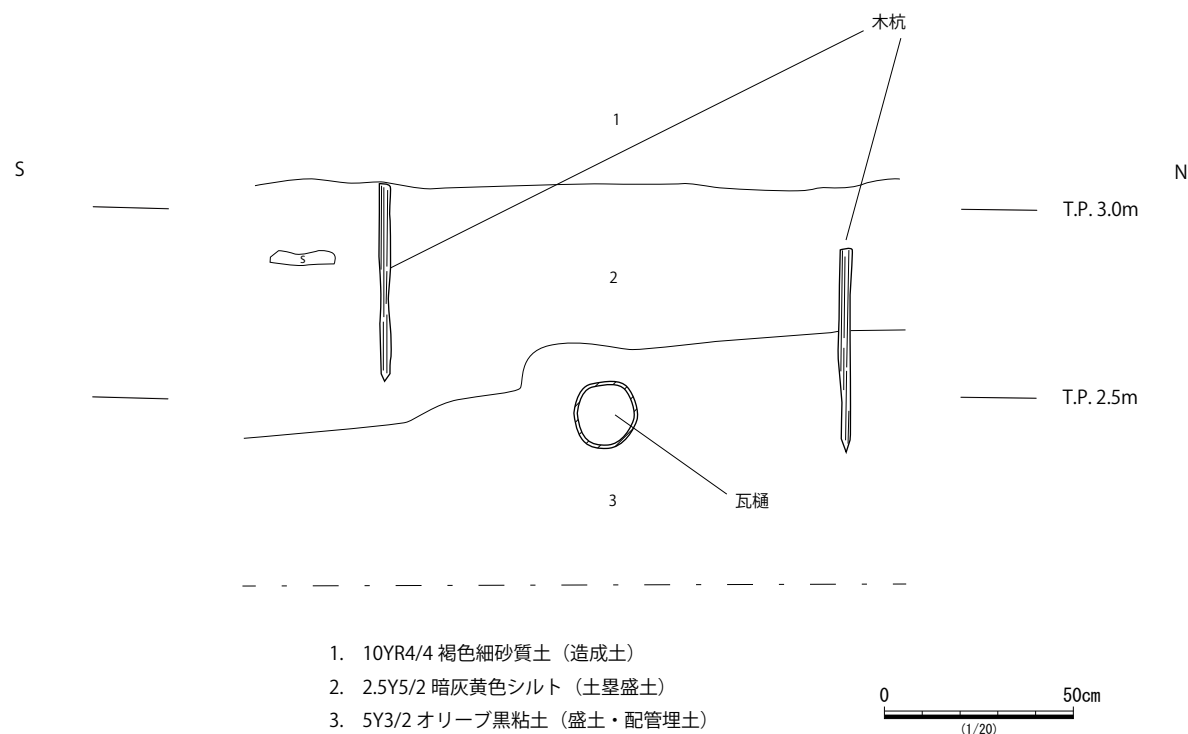
図3 瓦樋断面図 (1/20)
