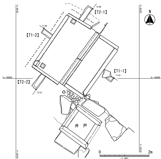
図3 薬医門基壇とトレンチ配置 (1/80)
