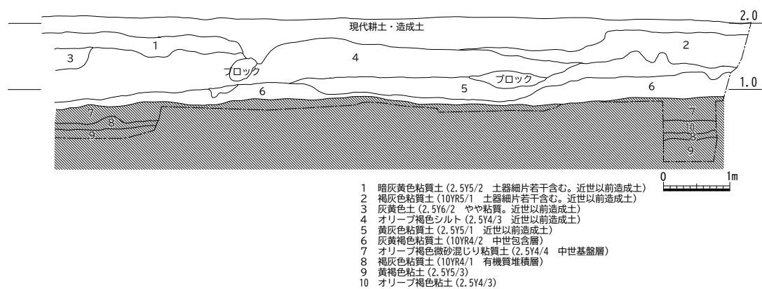
図3 断面図 (S = 1/80)
