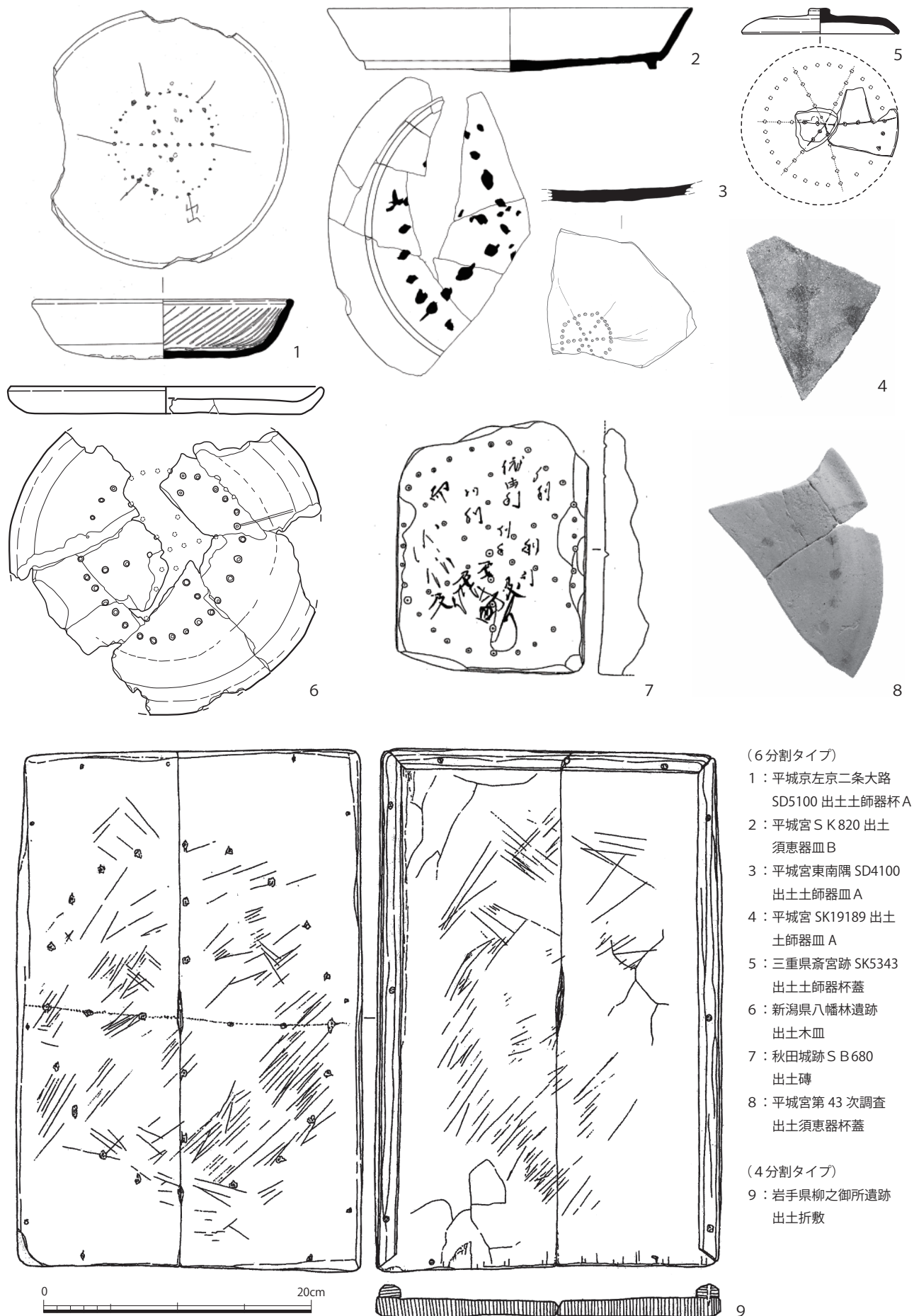
図4 出土かりうち盤 1:4
