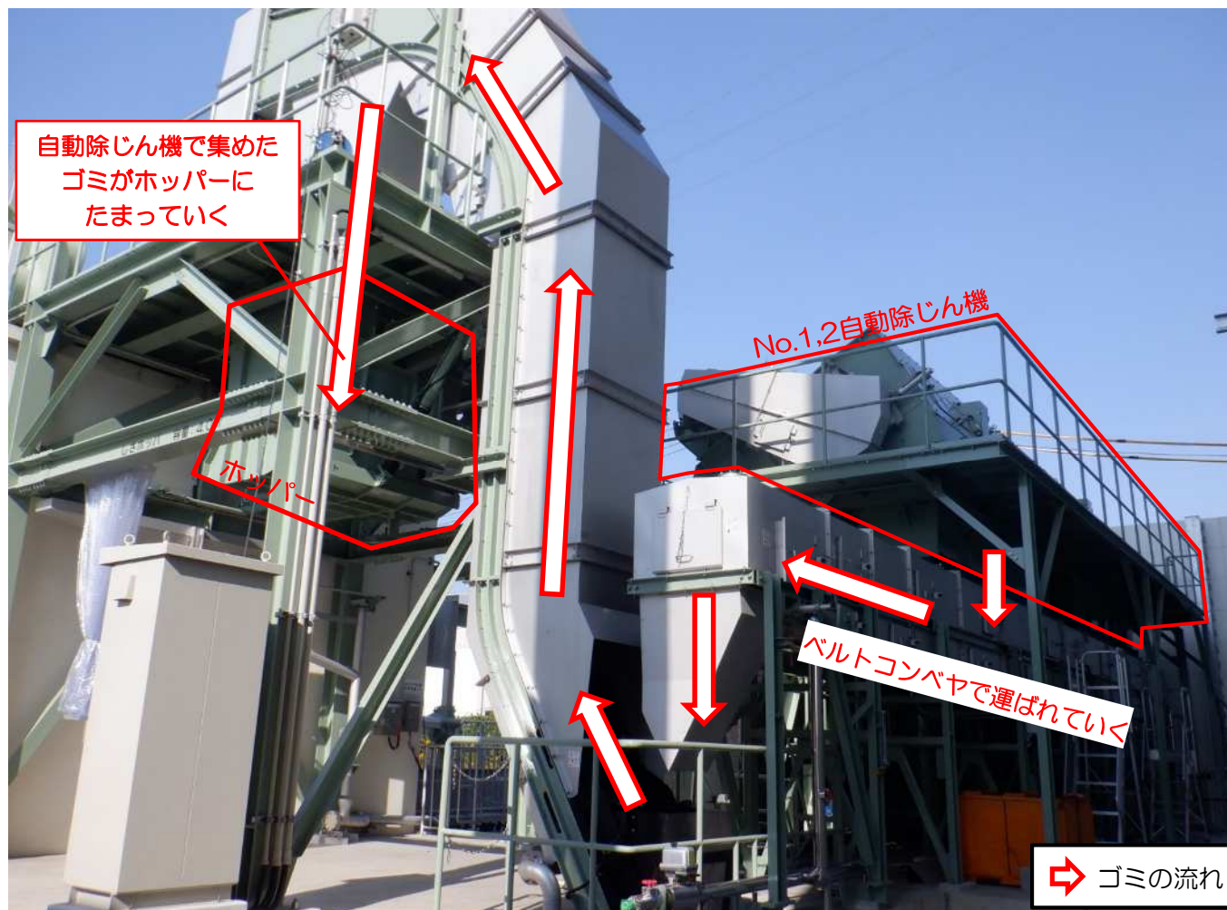
自動除じん機で集めたゴミの流れ
