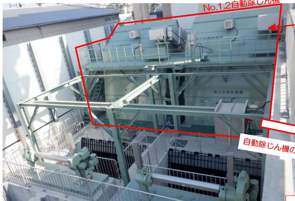
自動除じん機 上部
