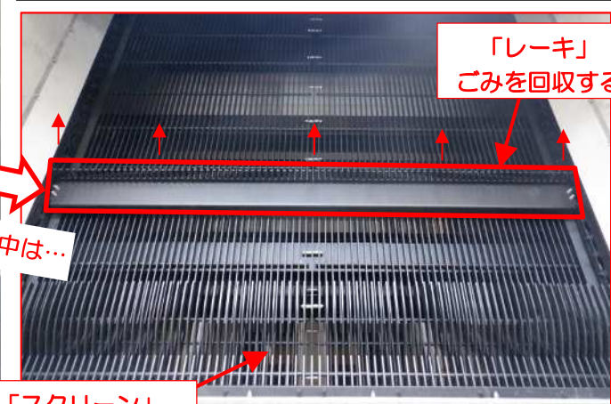
自動除じん機 下部
