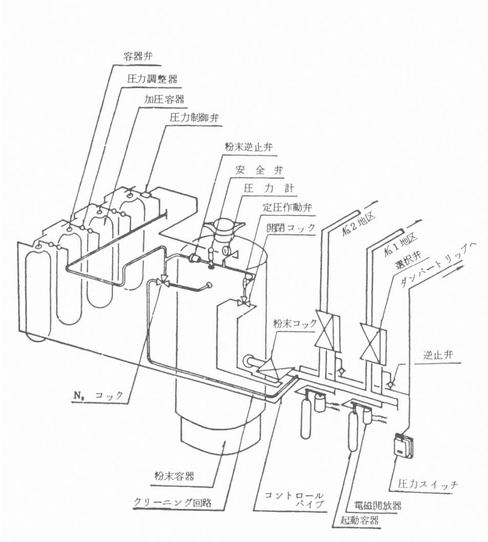
図8-2 粉末消火設備粉末容器附属機器図例
