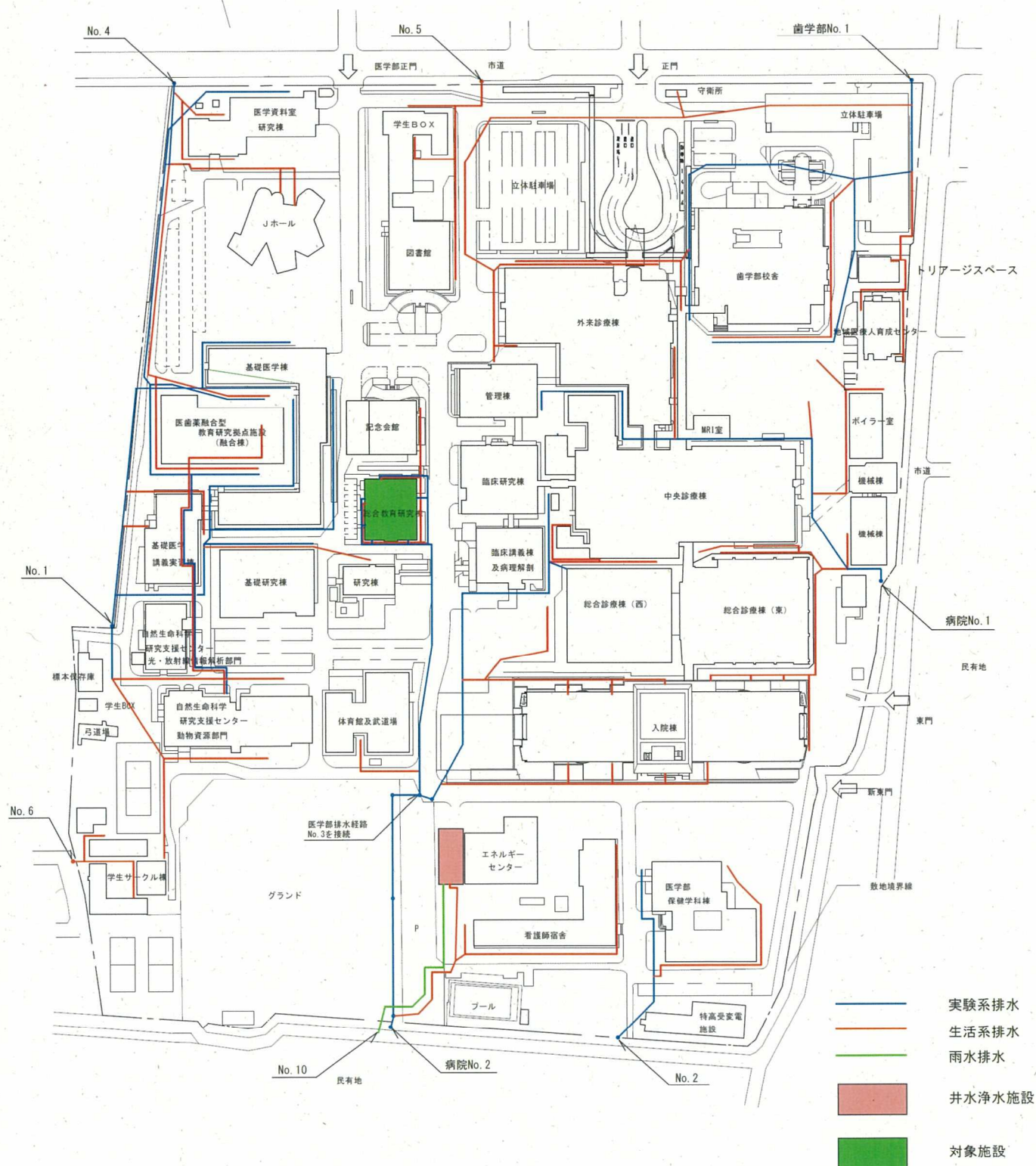
鹿 田 配 置 図
