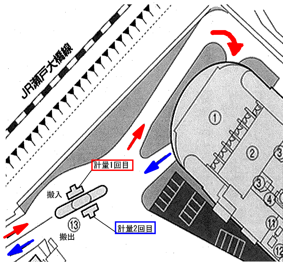
① プラットホーム ⑬ 計量棟
