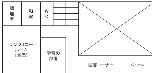
【2階平面図】
