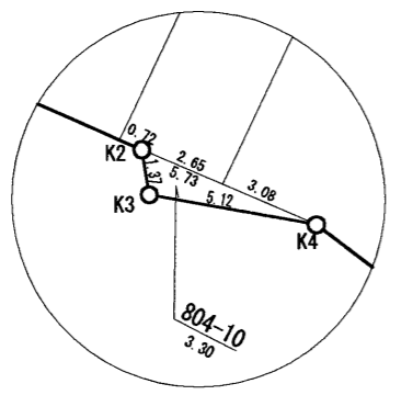
放大圖 S=1:250
