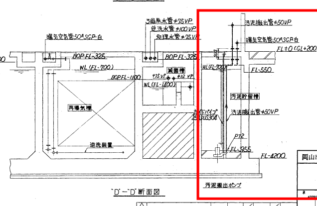
“D-D”断面図
