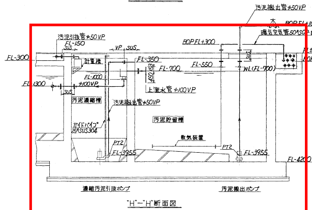
“H-H”断面図
