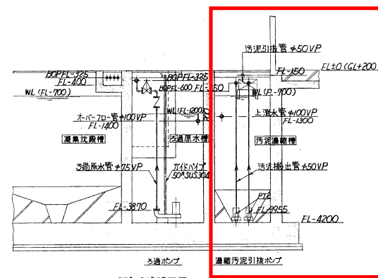
“B-B”断面図
