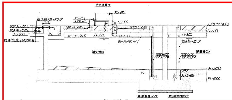
“A-A”断面図
