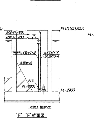
“F-F”断面図
