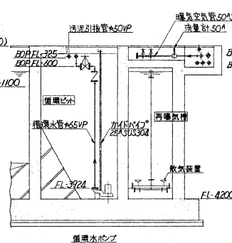
“E-E”断面図
