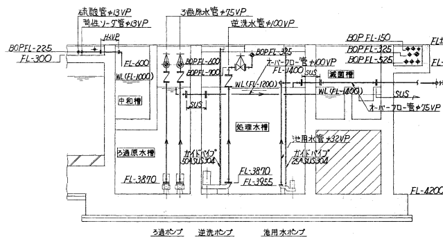
“G-G”断面図
