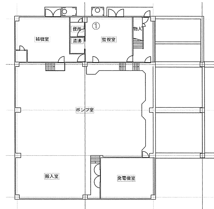
[ 1階 ]
