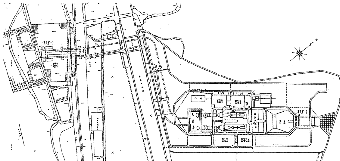
【平田ポンプ場 一般平面図】
