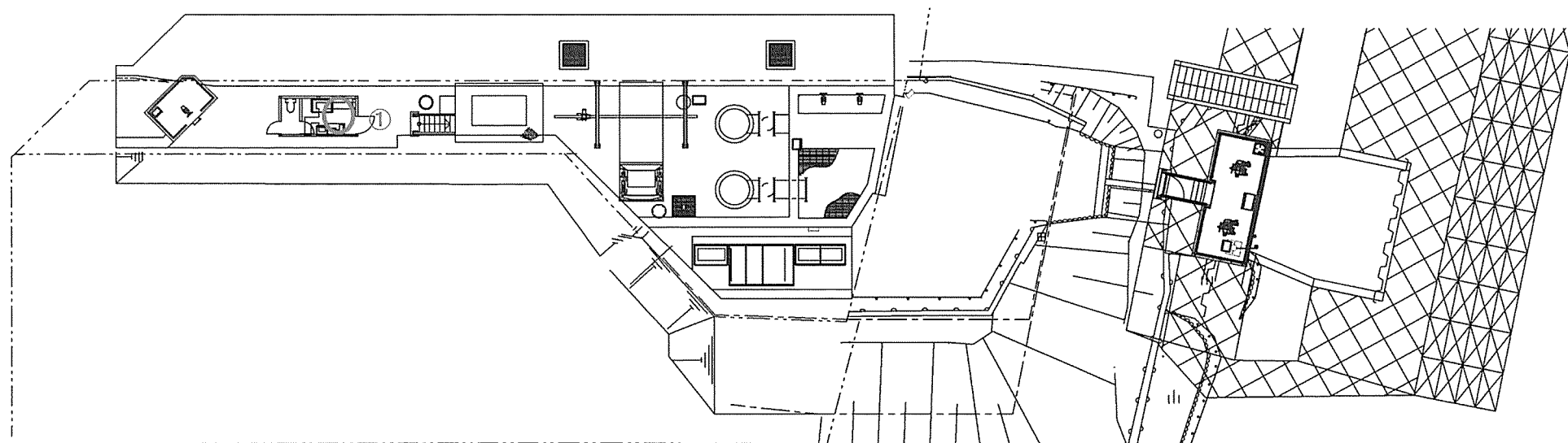
〔北長瀬ポンプ場 一般平面図〕
