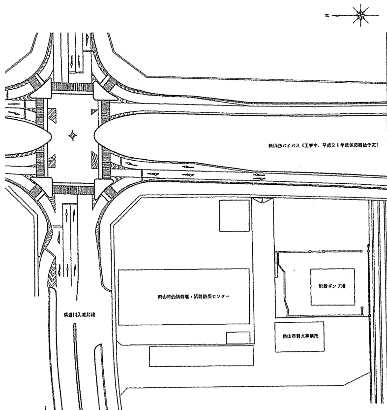
[ 野殿ポンプ場 一般平面図 ]
