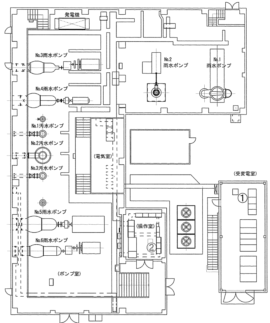
[ ポンプ室 ]
