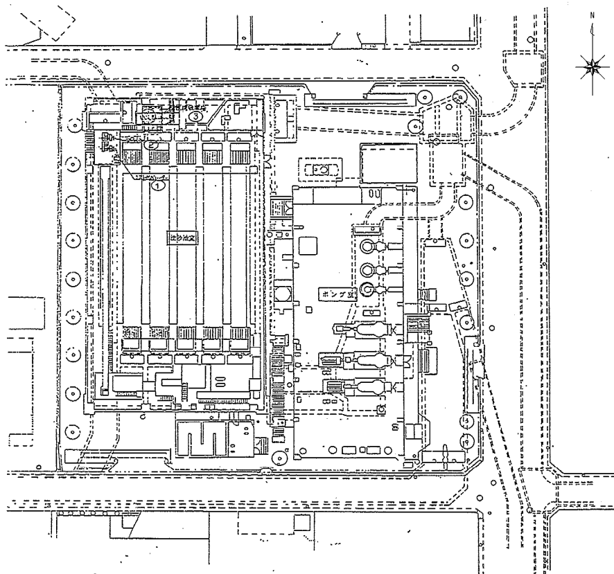
[ 巖井ポンプ場 一般平面図 ]
