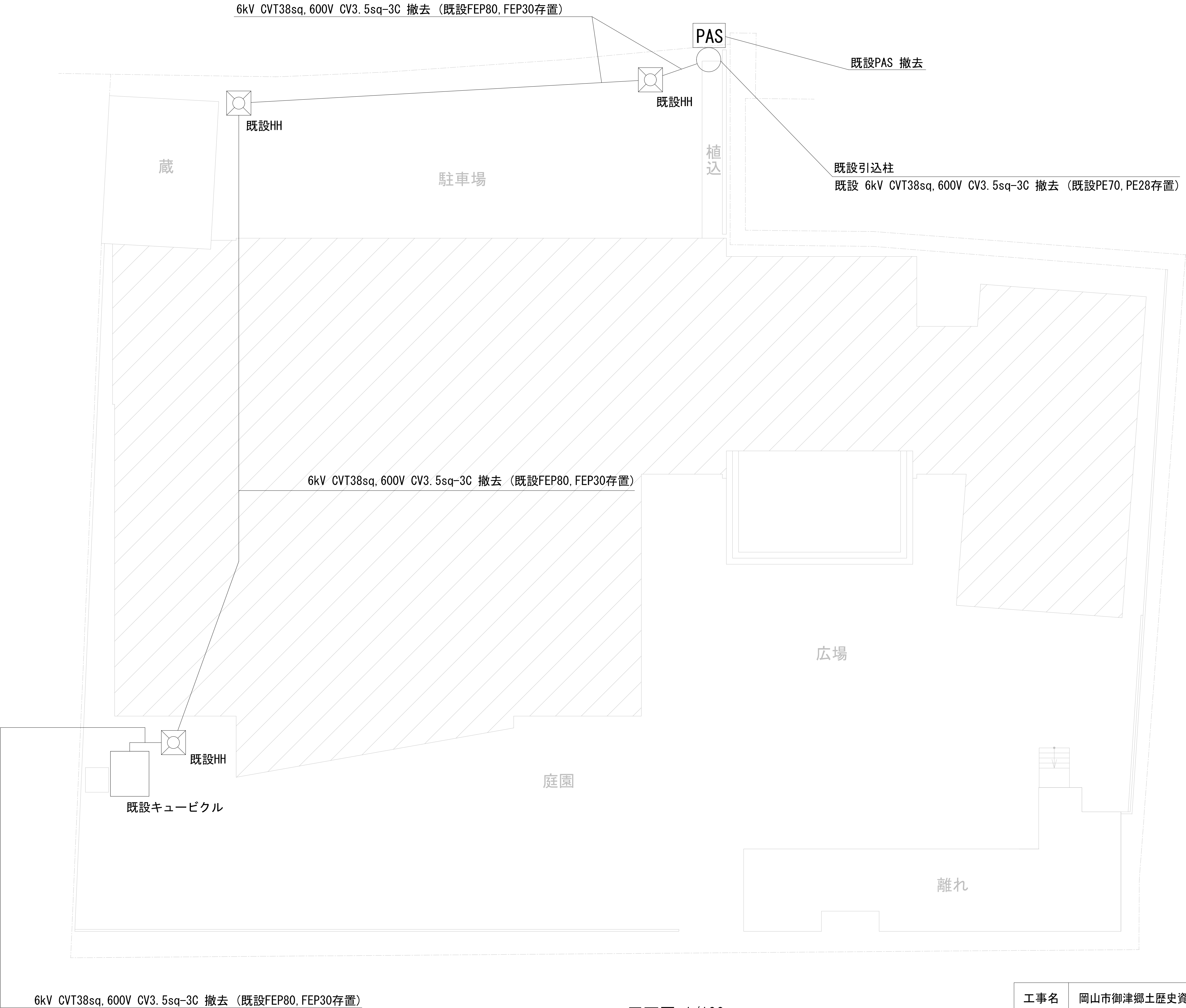
平面図 1/100
