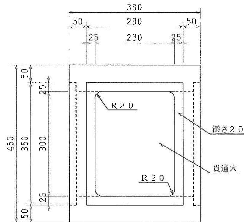
火袋詳細図
