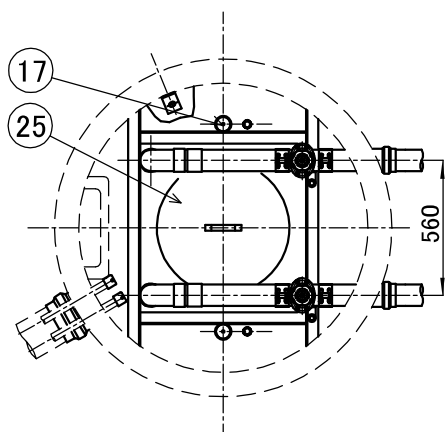
A-A矢視図
