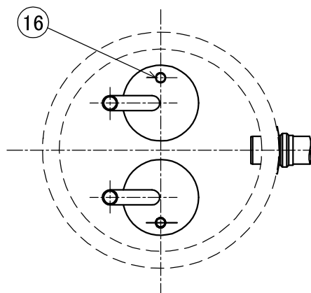
B-B矢視図
