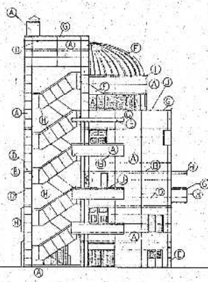
南立面圖 1:200
