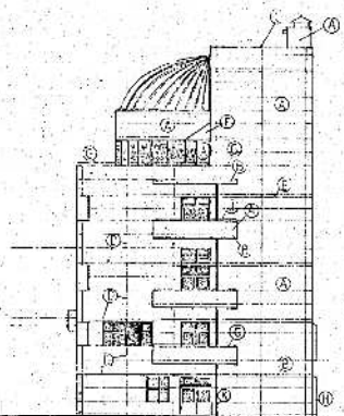
北立面圖 1:200
