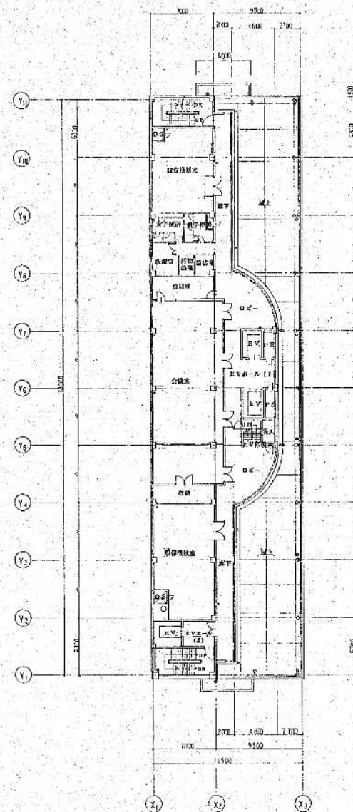
5 附平面图 1:200
