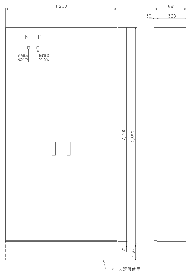
【盤更新】 昇降床制御盤 S=1:20(A3) 面 数：1面
