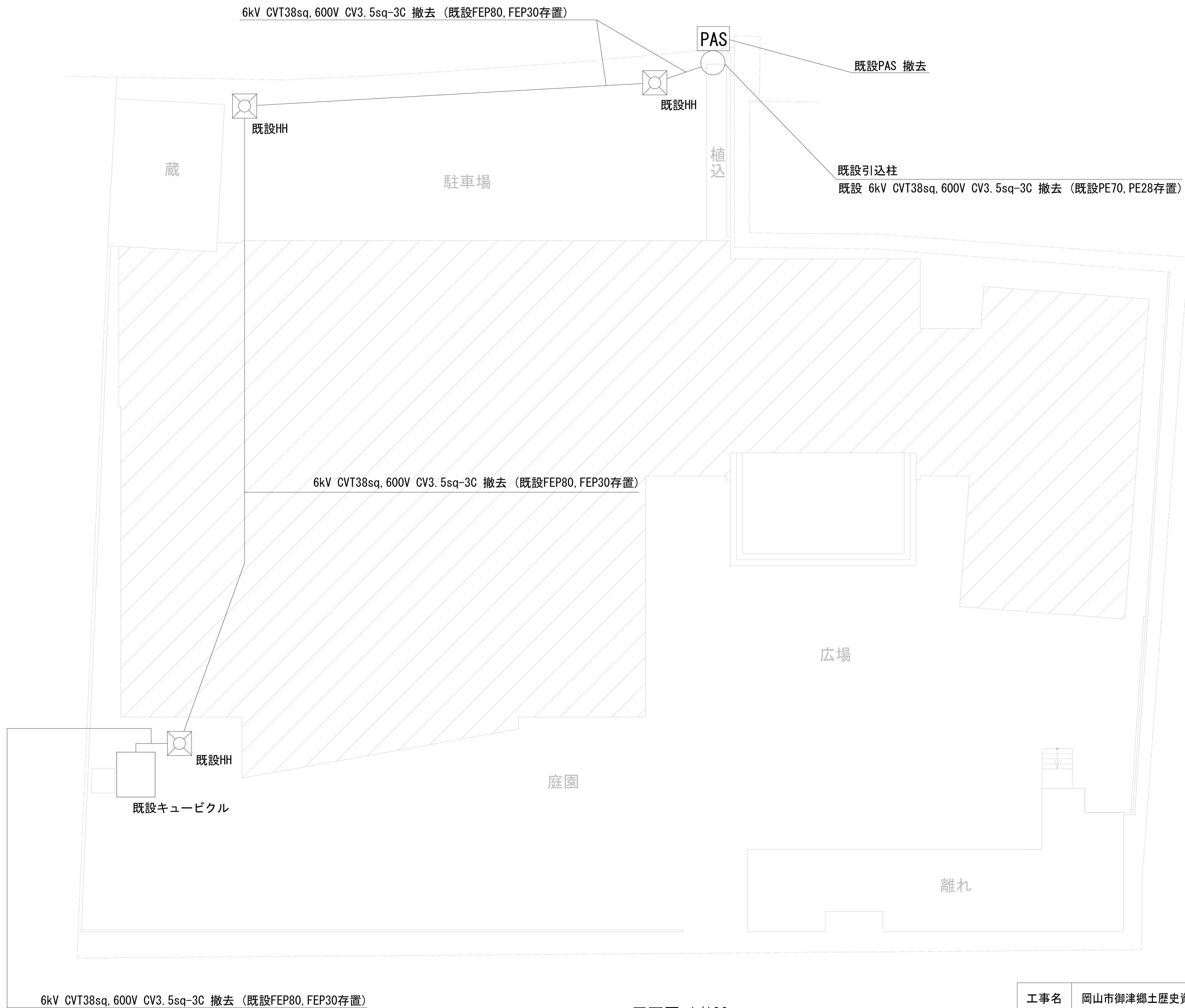
平面図 1/100
