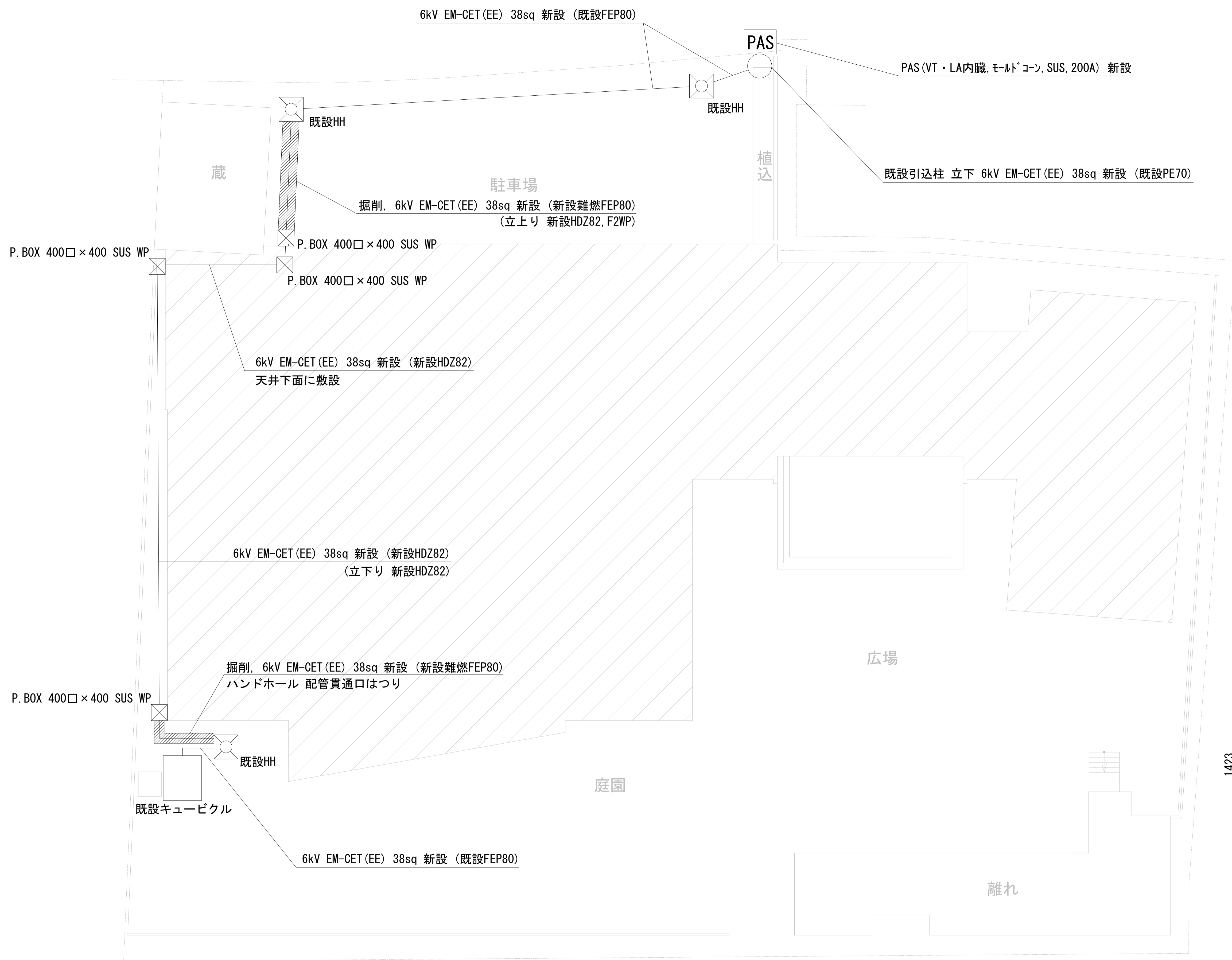
平面図 1/100
