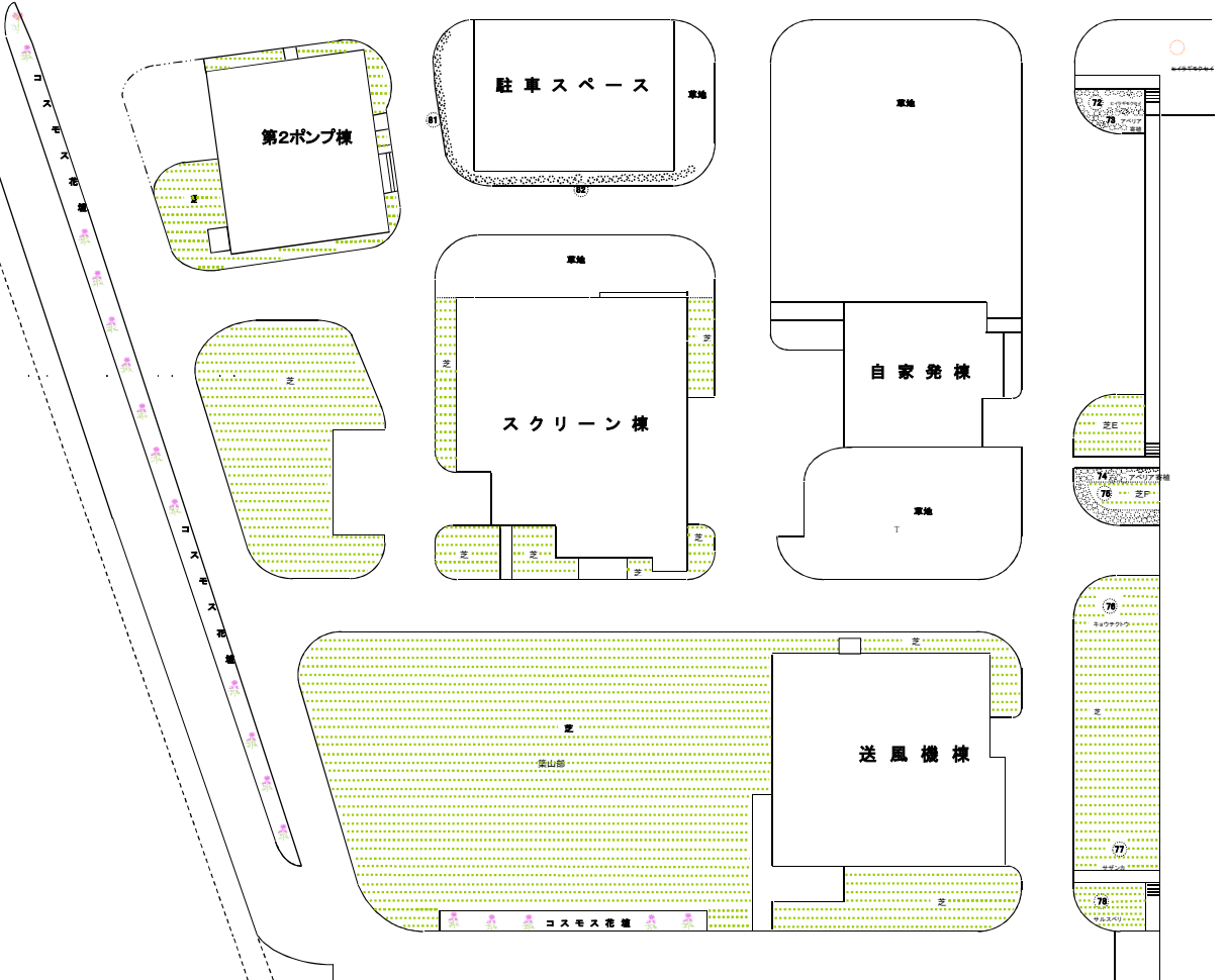
岡東浄化センター正門廻り植栽図
