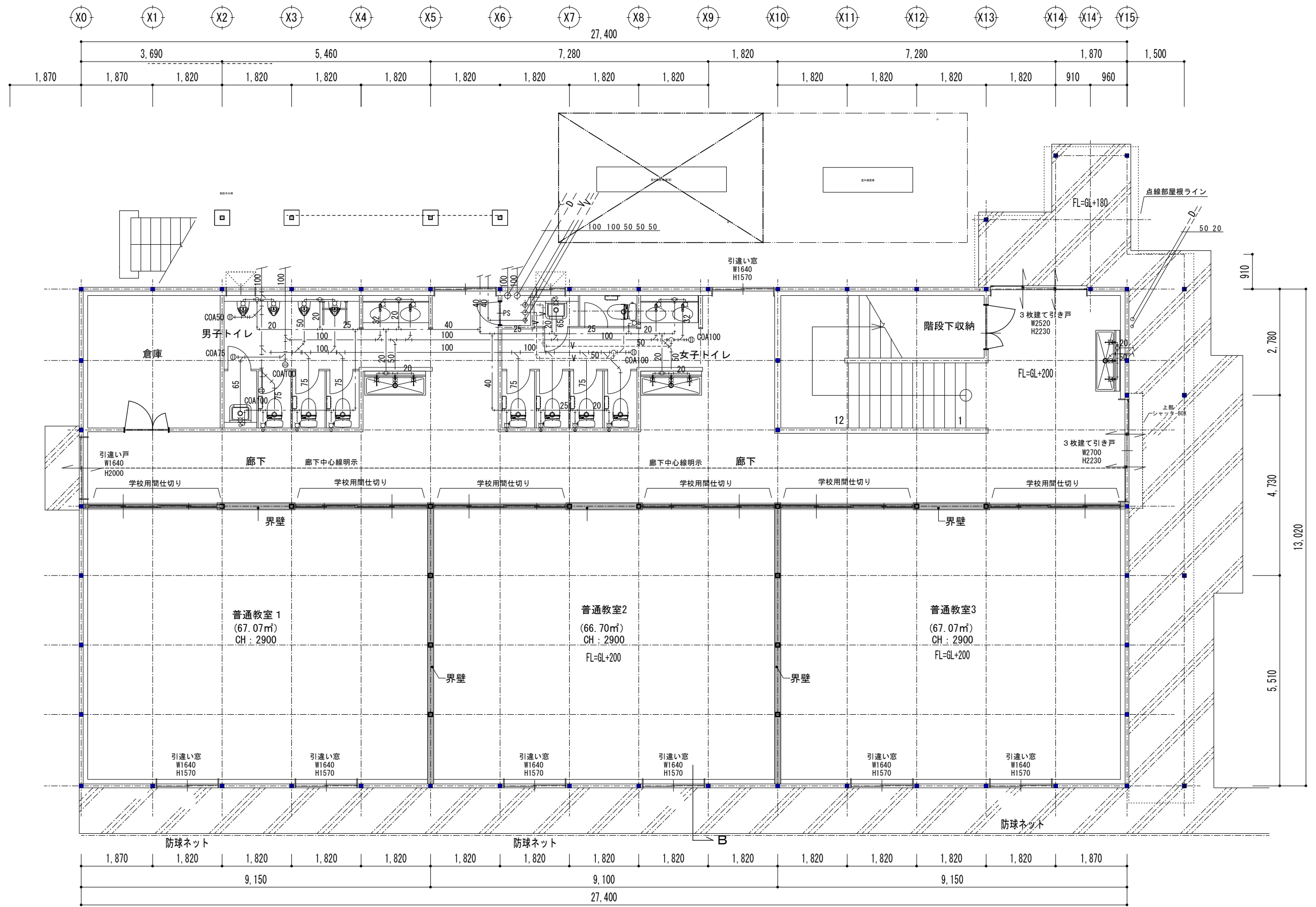
1階平面図 1/100
