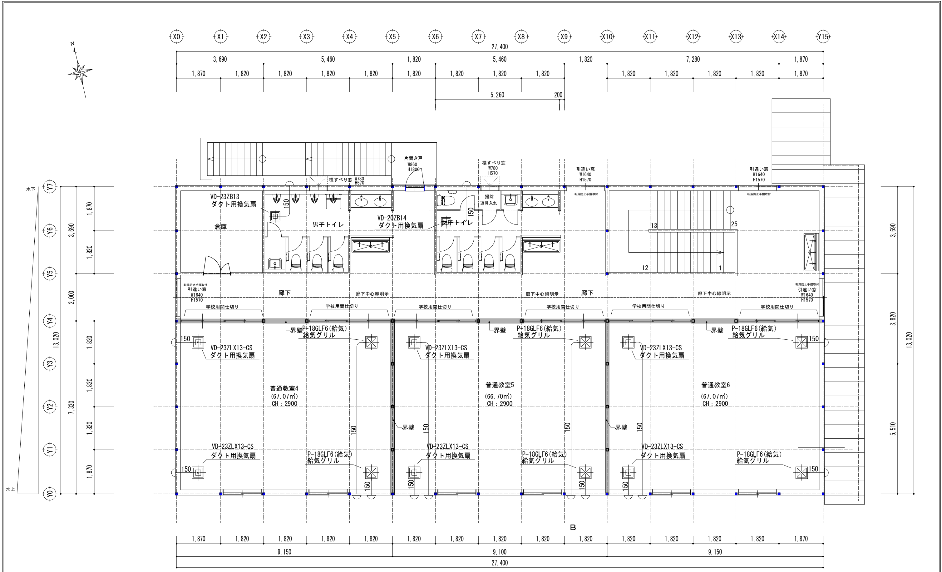
2階平面図 1/100
