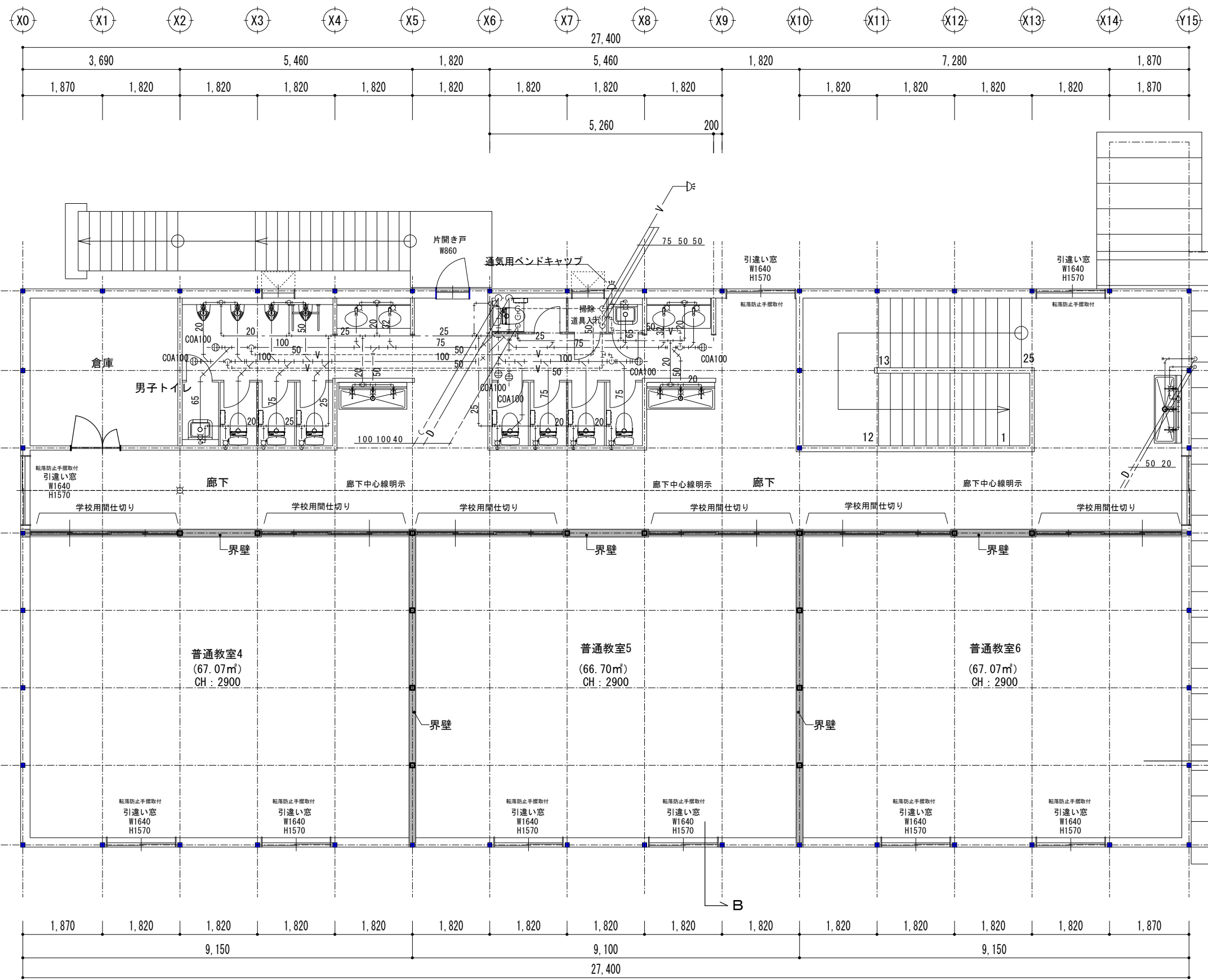
2階平面図 1/100
