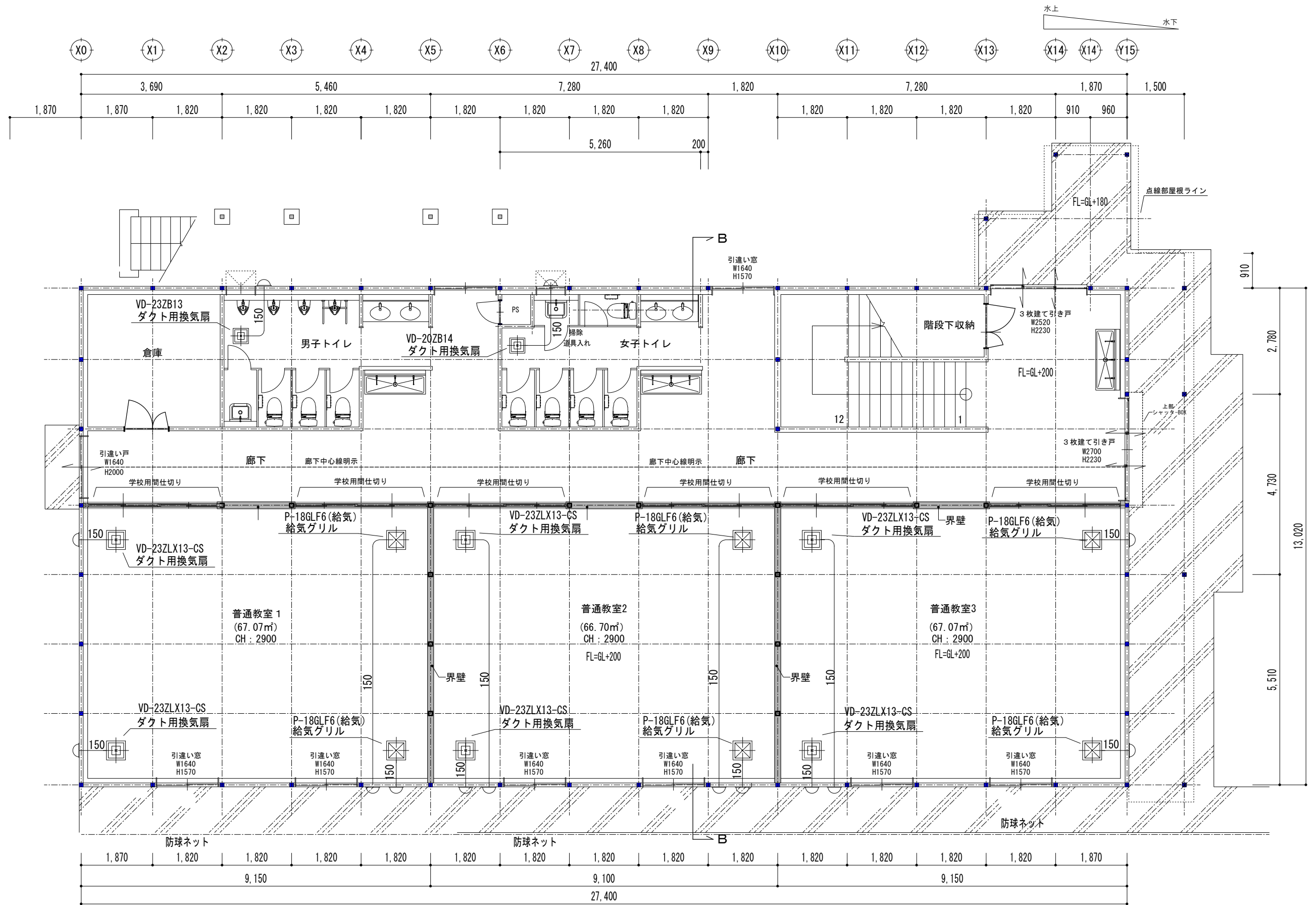
1階平面図 1/100
