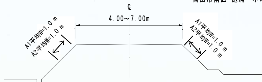
標準横断面図 S=1:100
