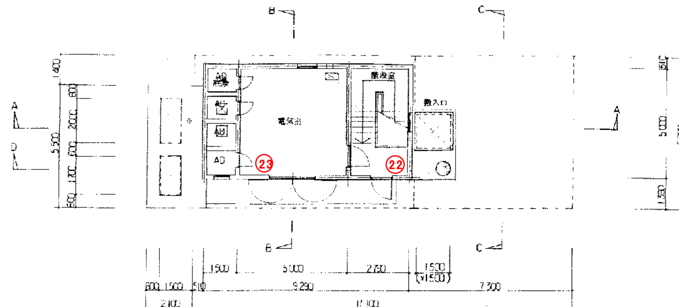
1F 平面図 1/100
