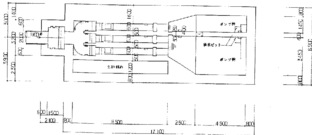
B3F 平面図 1/100
