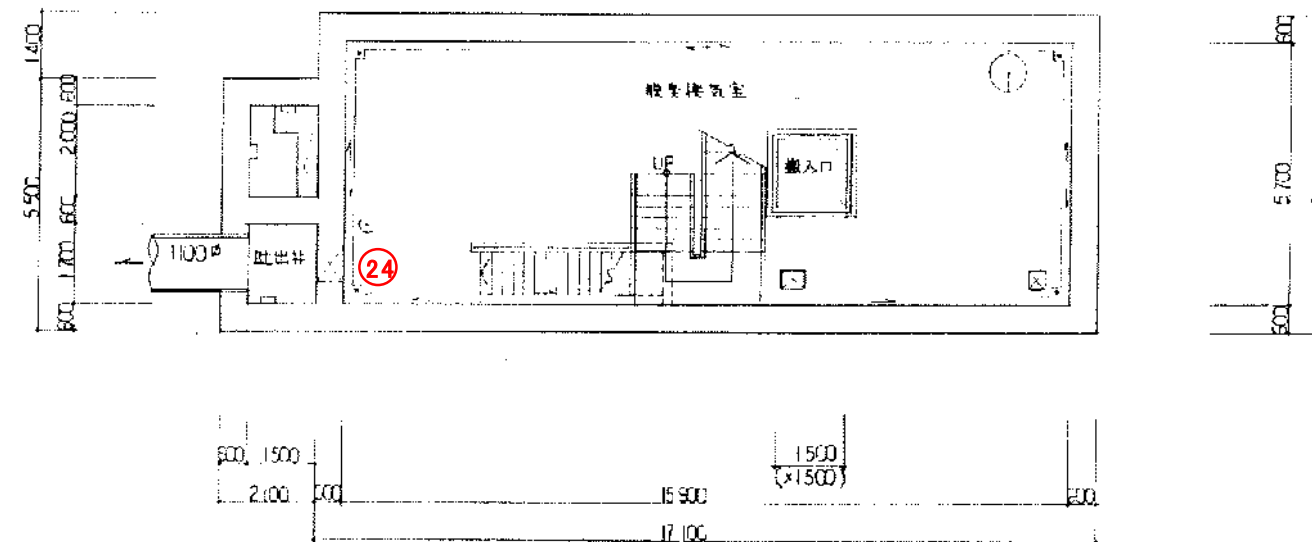
B1F 平面図 1/100
