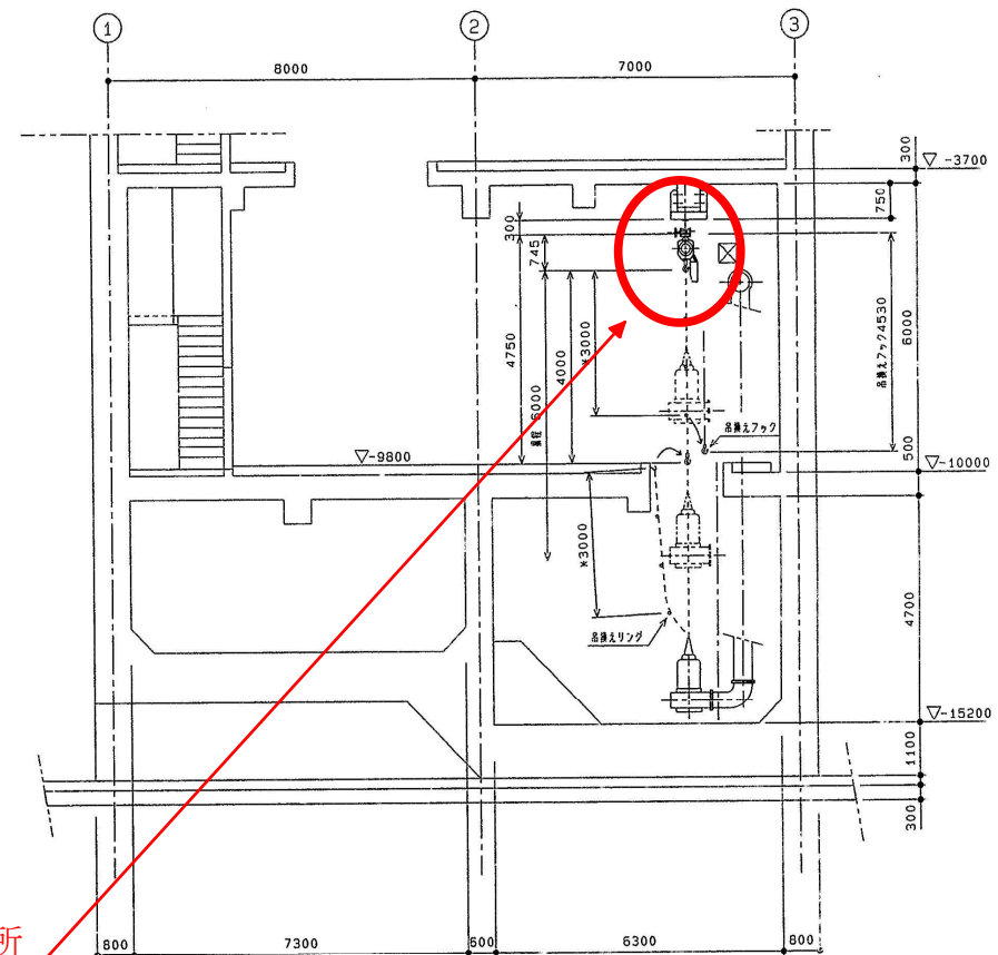
A-A 断面図
