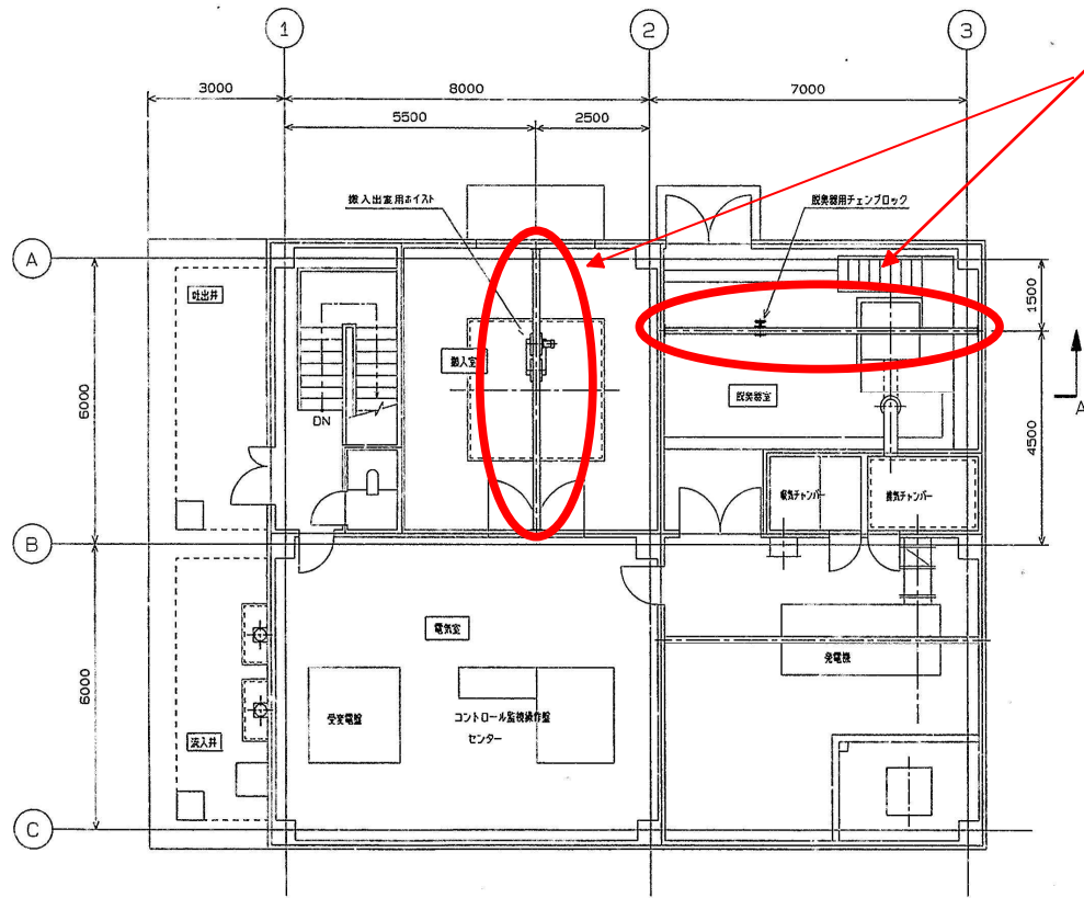
1FL 平面図
