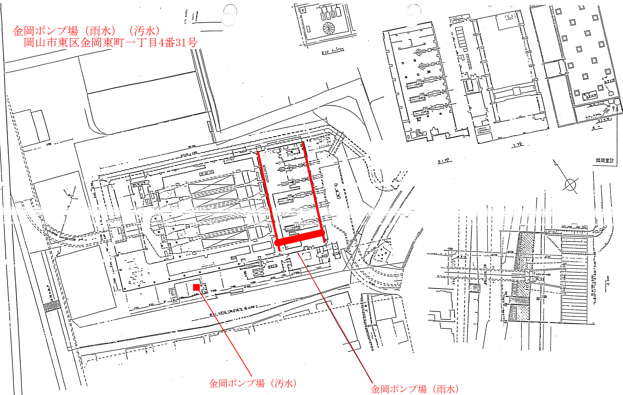
金岡ポンプ場平面図
