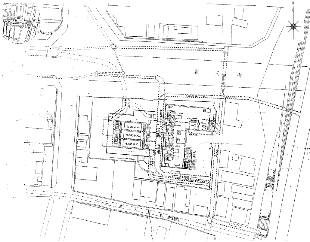
[ 天瀬ポンプ場 一般平面図 ]
