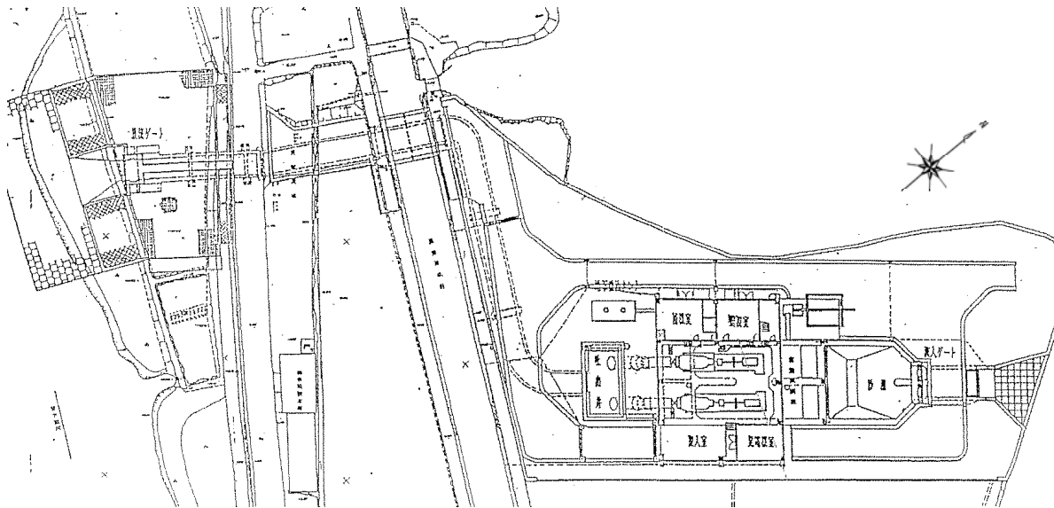
【平田ポンプ場 一般平面図】
