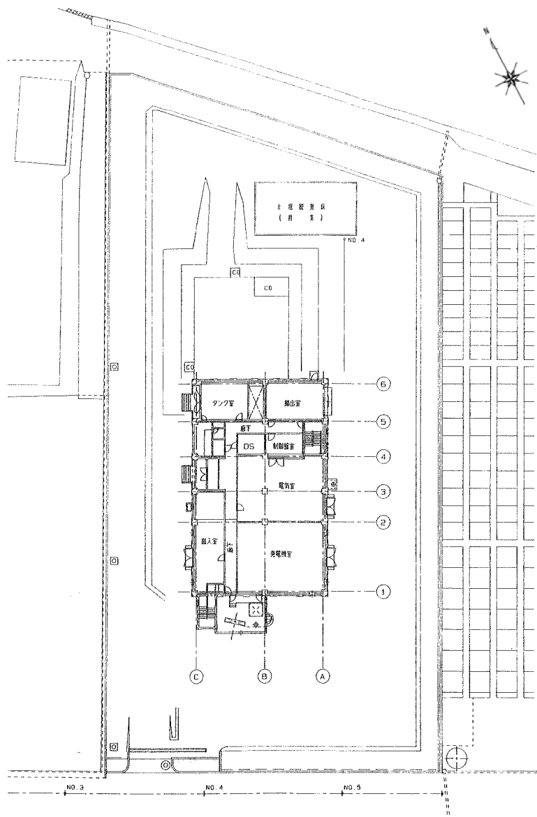
[ 錦ポンプ場 一般平面図 ]
