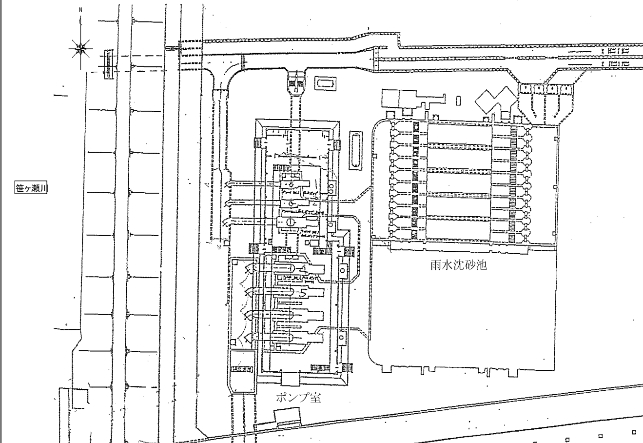
【笹ヶ瀬ポンプ場 一般平面図】
