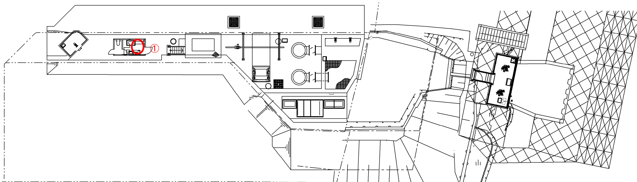
[ 北長瀬ポンプ場 一般平面図 ]
