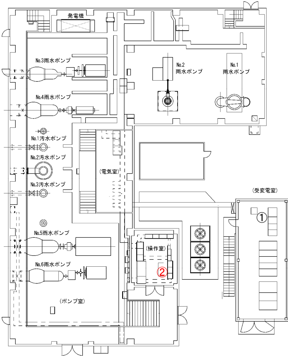
[ ポンプ室 ]
