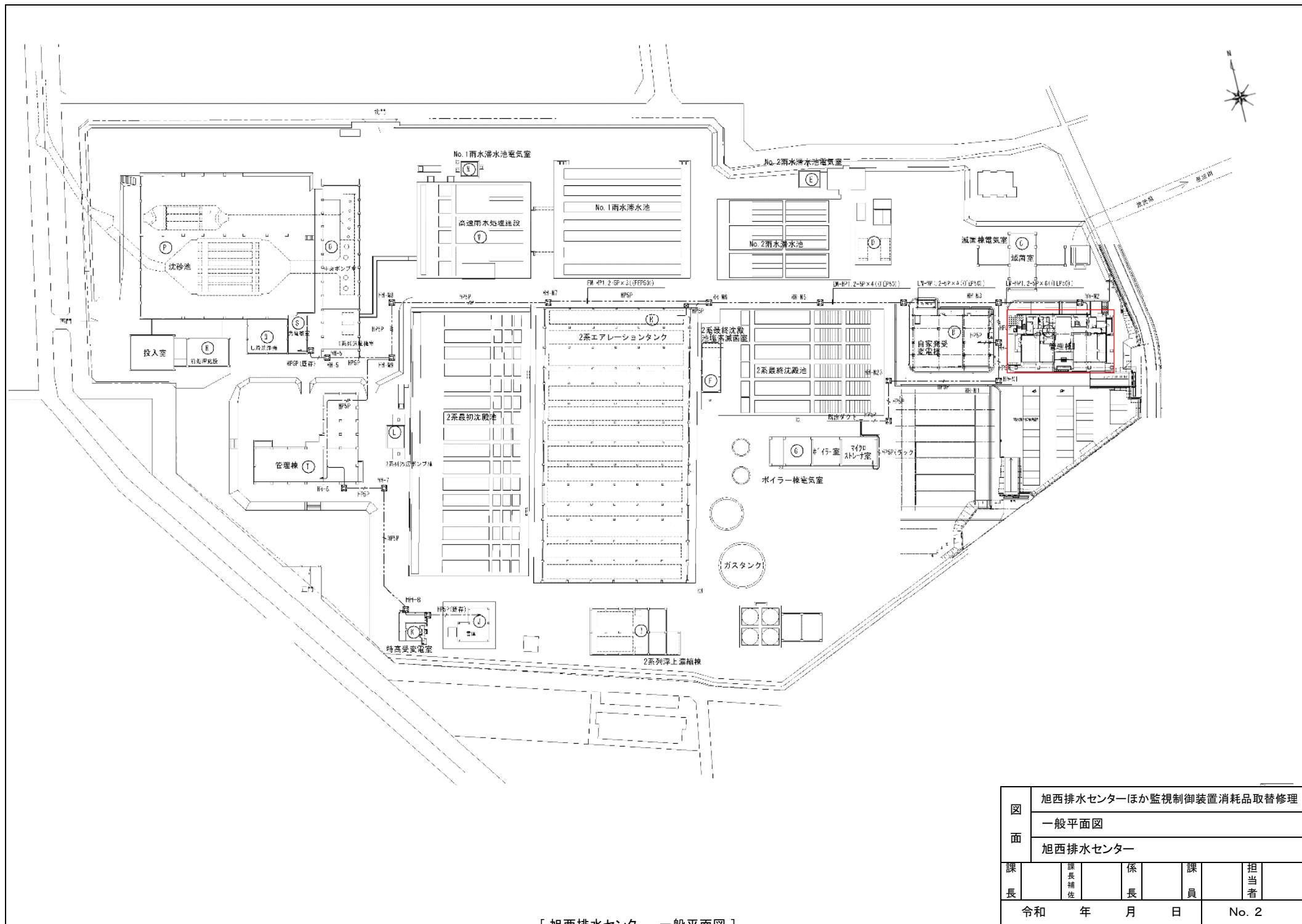
「旭西排水センター 一般平面図」
