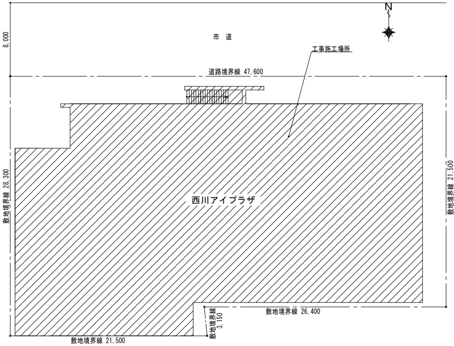
配置図 S:1/200
