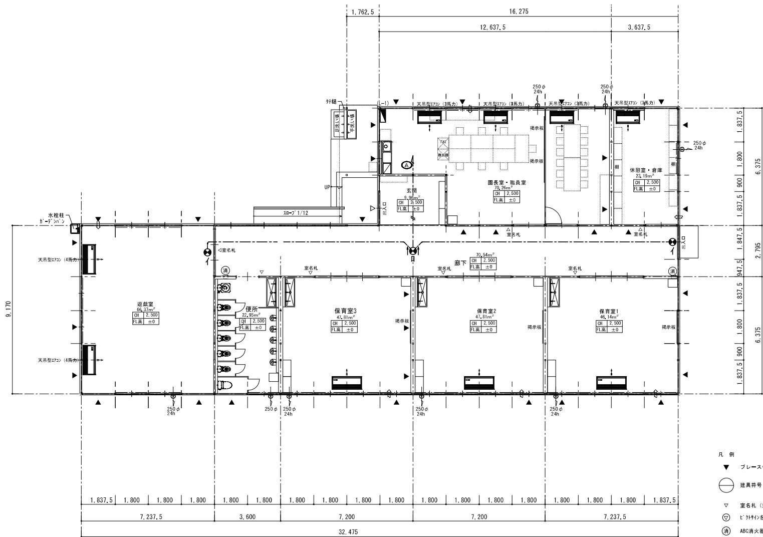
平面図 1/100 底 1階床面積：401.55㎡ + 11.24㎡ = 412.79㎡
