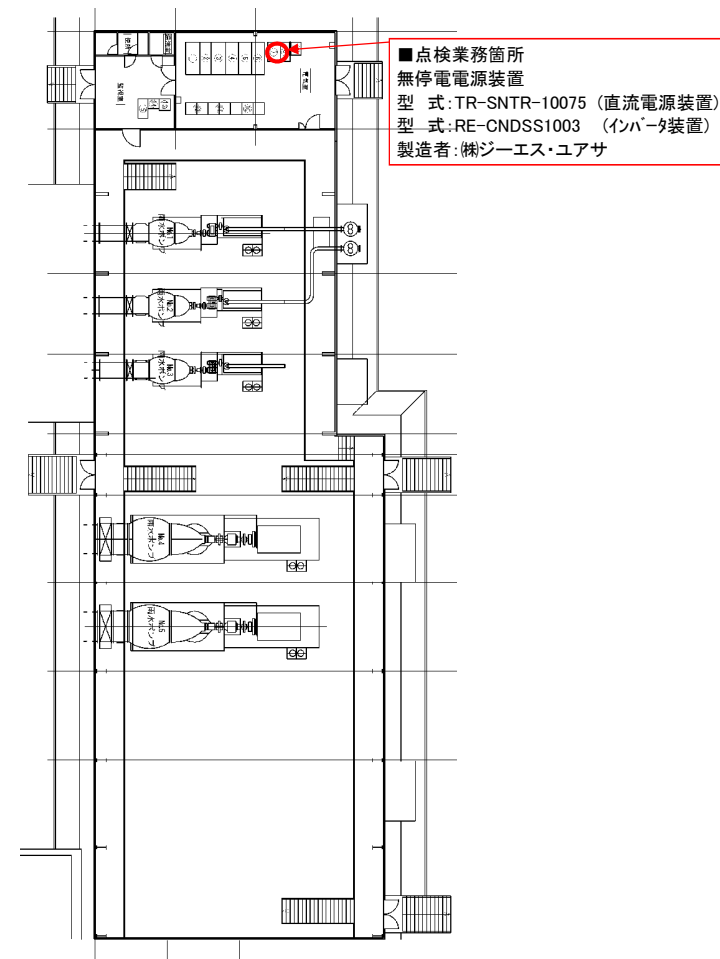
[ ポンプ室平面図 ]
