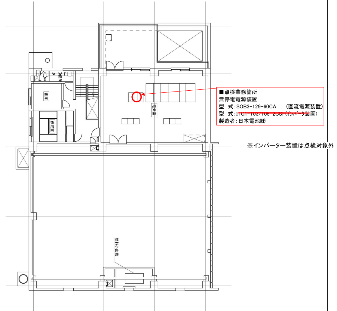
[ ポンプ室平面図 ]
