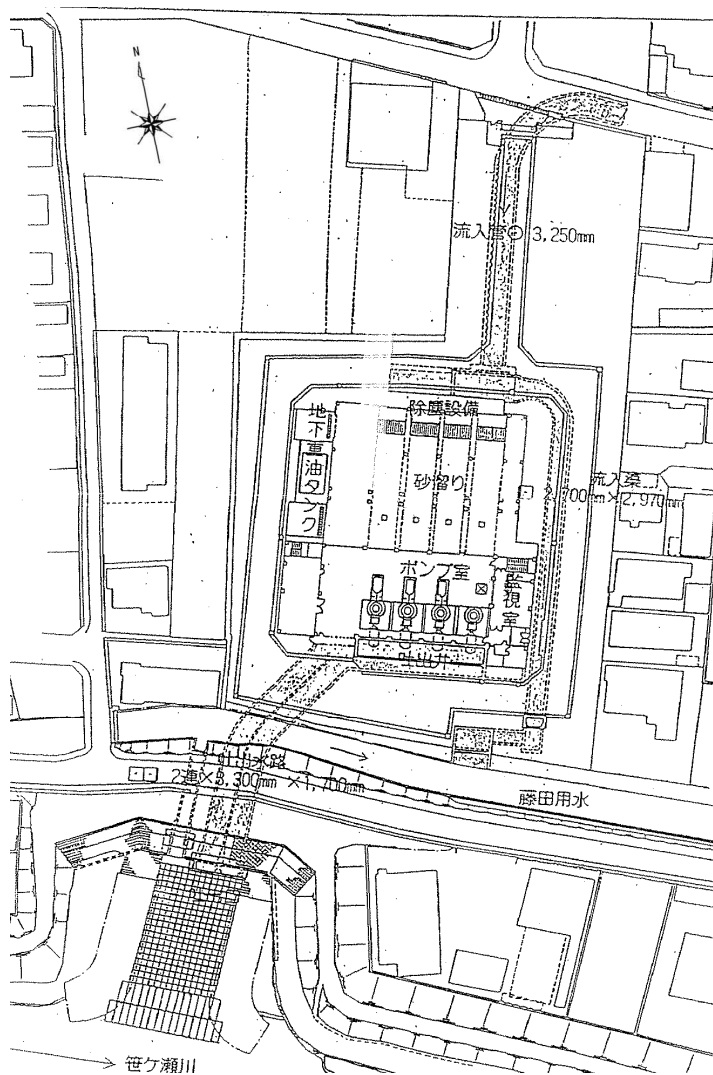
[ 当新田ポンプ場 一般平面図 ]
