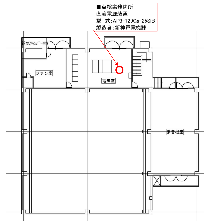
[ 2階平面図 ]
