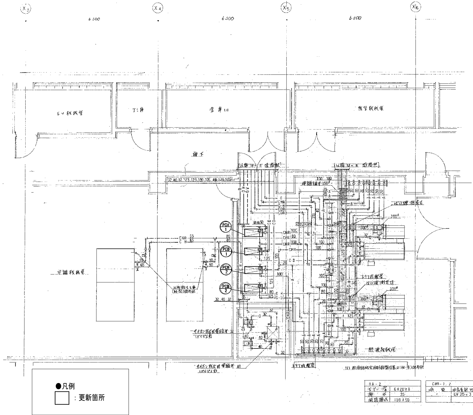
B2階 空調・熱源機械室 平面詳細図 (S=1/100)
