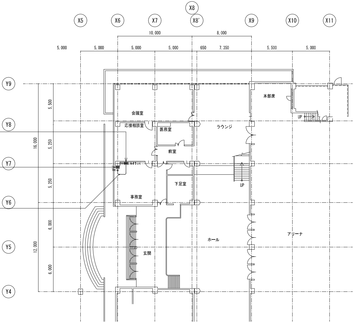
体育館（1階）平面図 【S=1:200】
