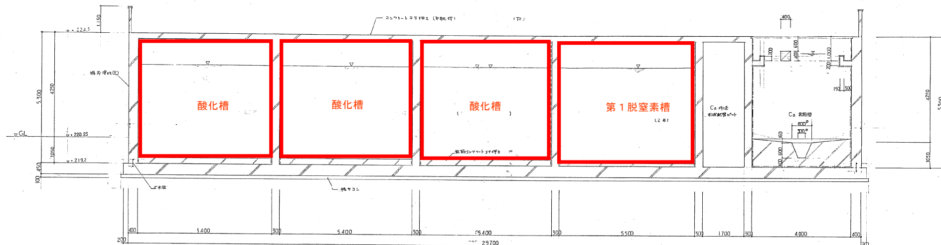
FC-D 断面図
