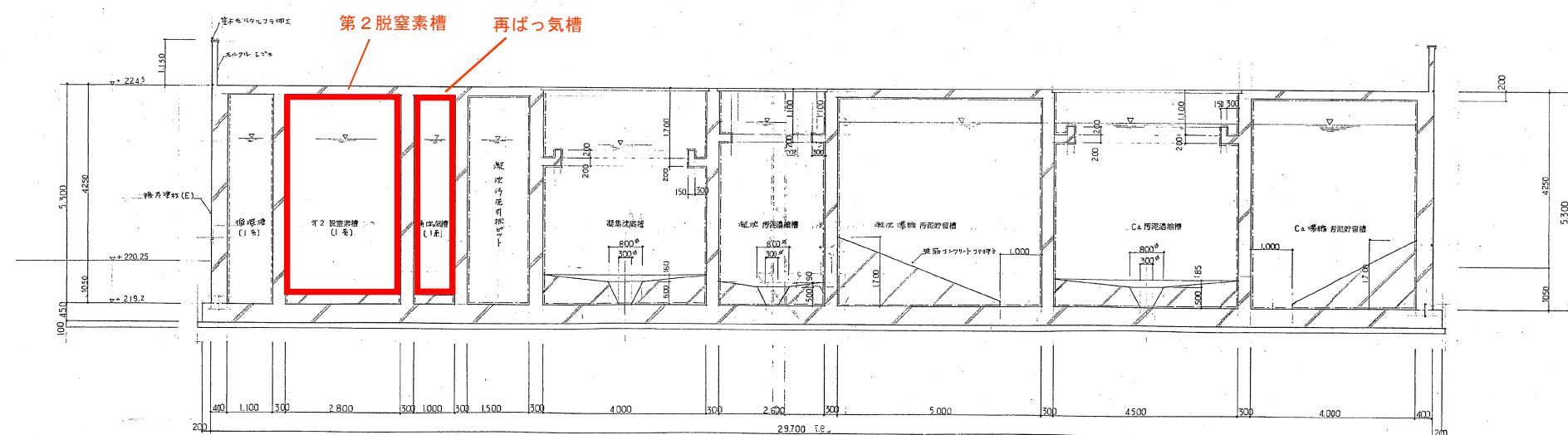
FC-D 断面図
