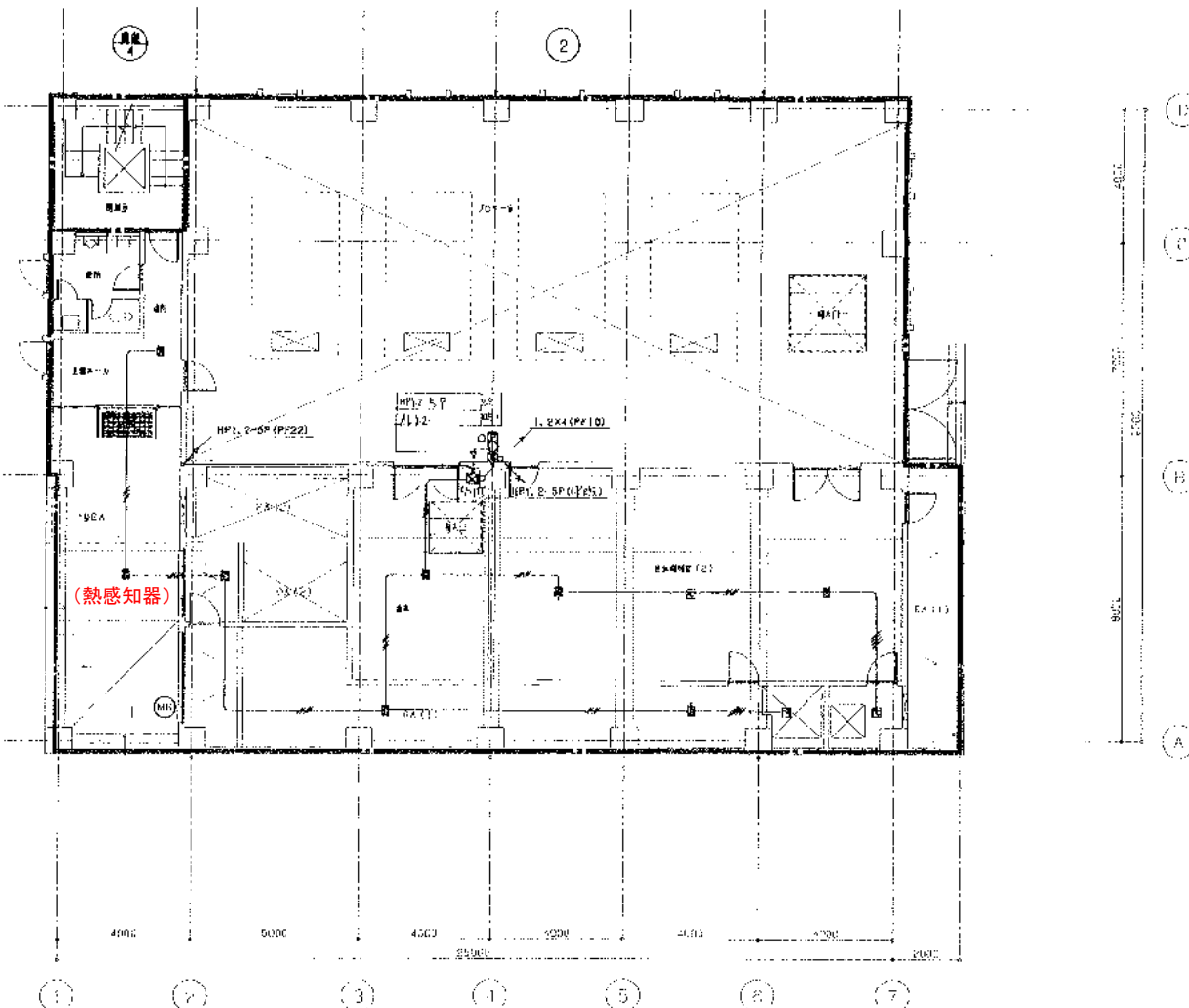
① 1F 平面図 1:100
