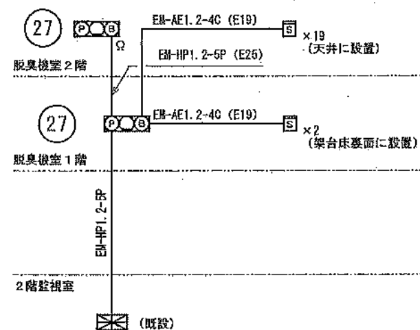
系統図
