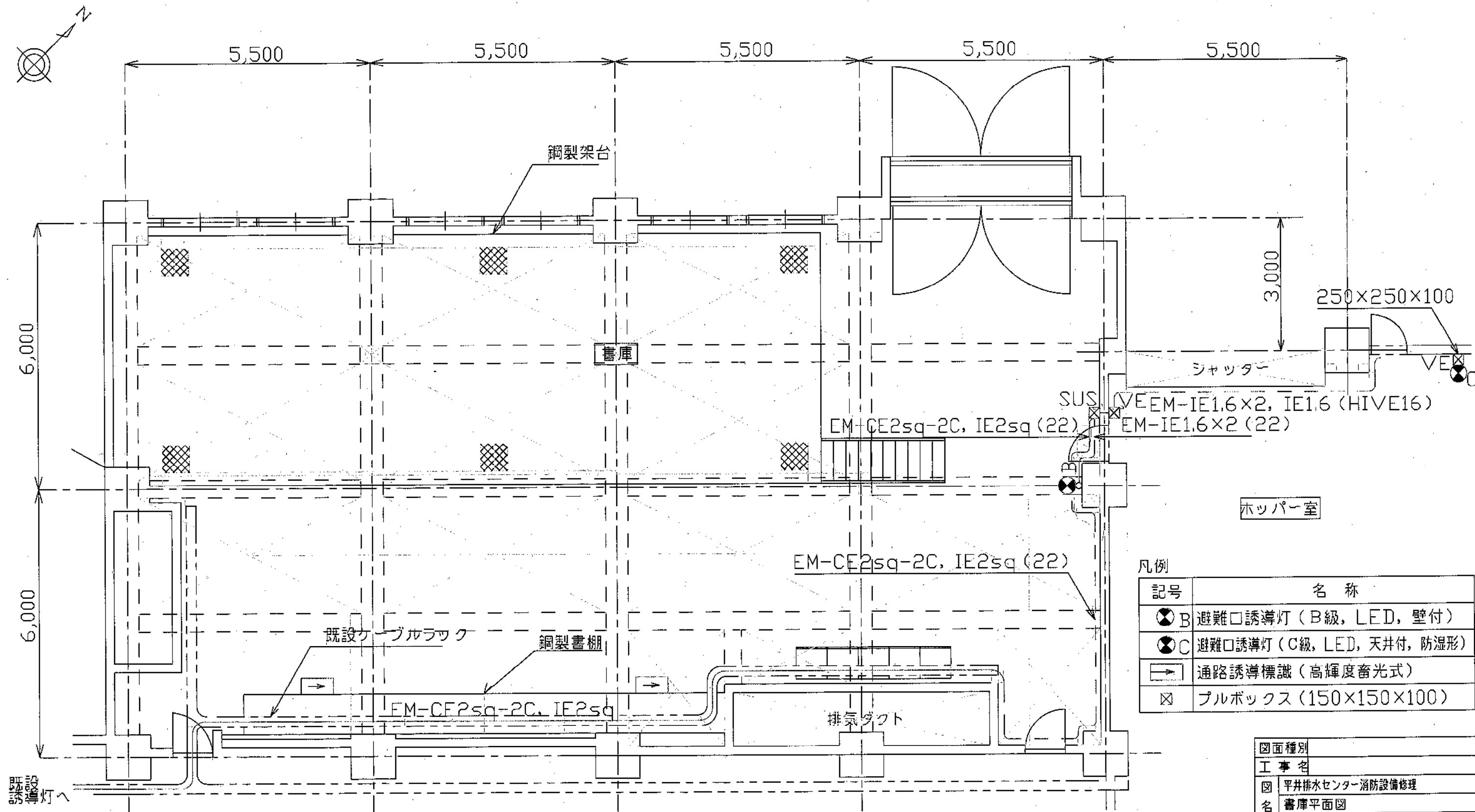
書庫平面図 S=1/120
