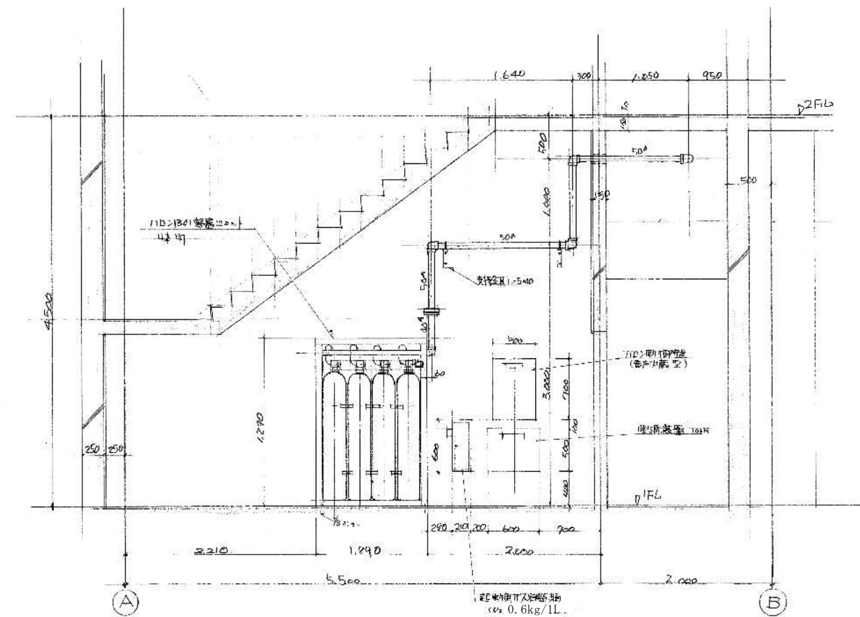
1-1 断面図 1/50
