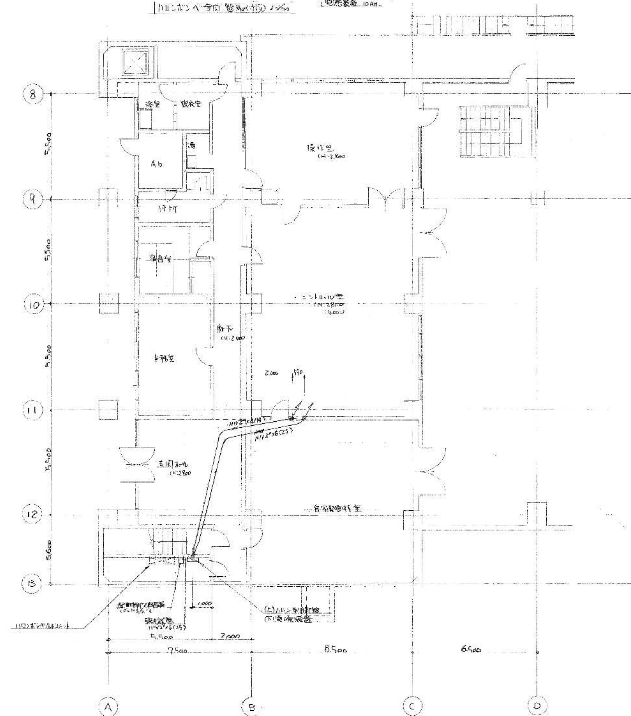
1階平面図 5/100
