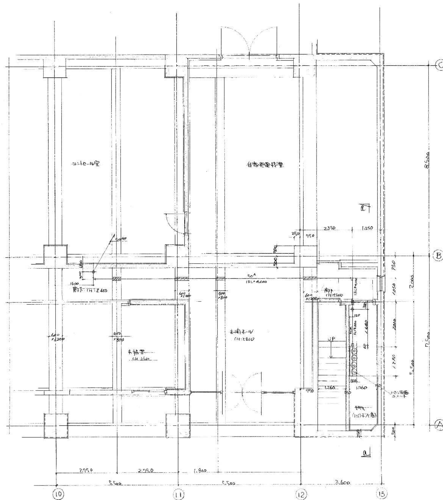
1階平面図 1/50
