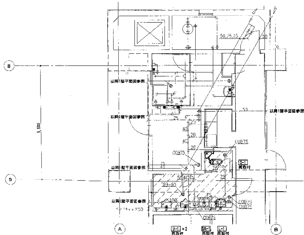
便所詳細図(改修) 1/50
