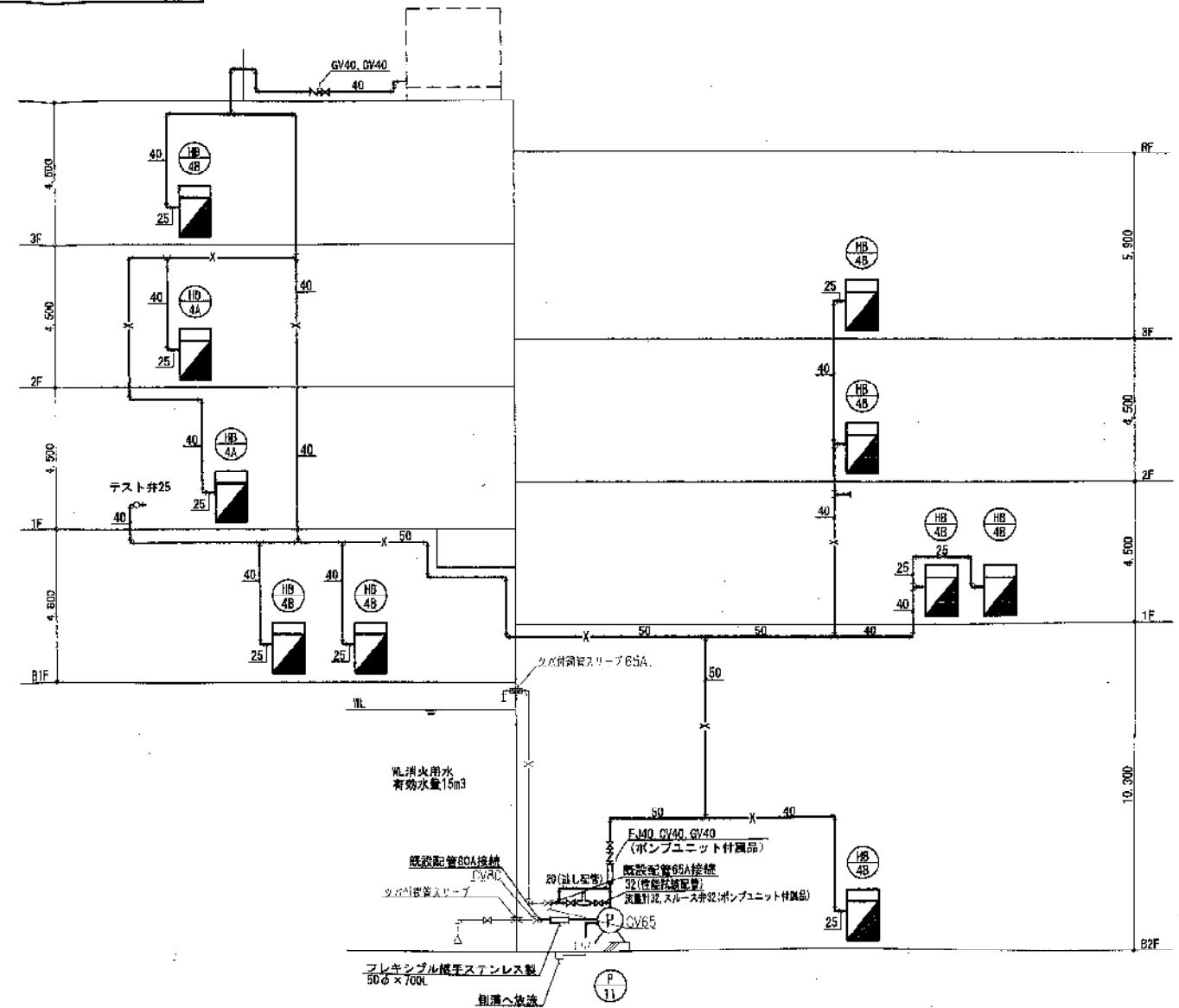
消火設備系統図 NO SCALE
