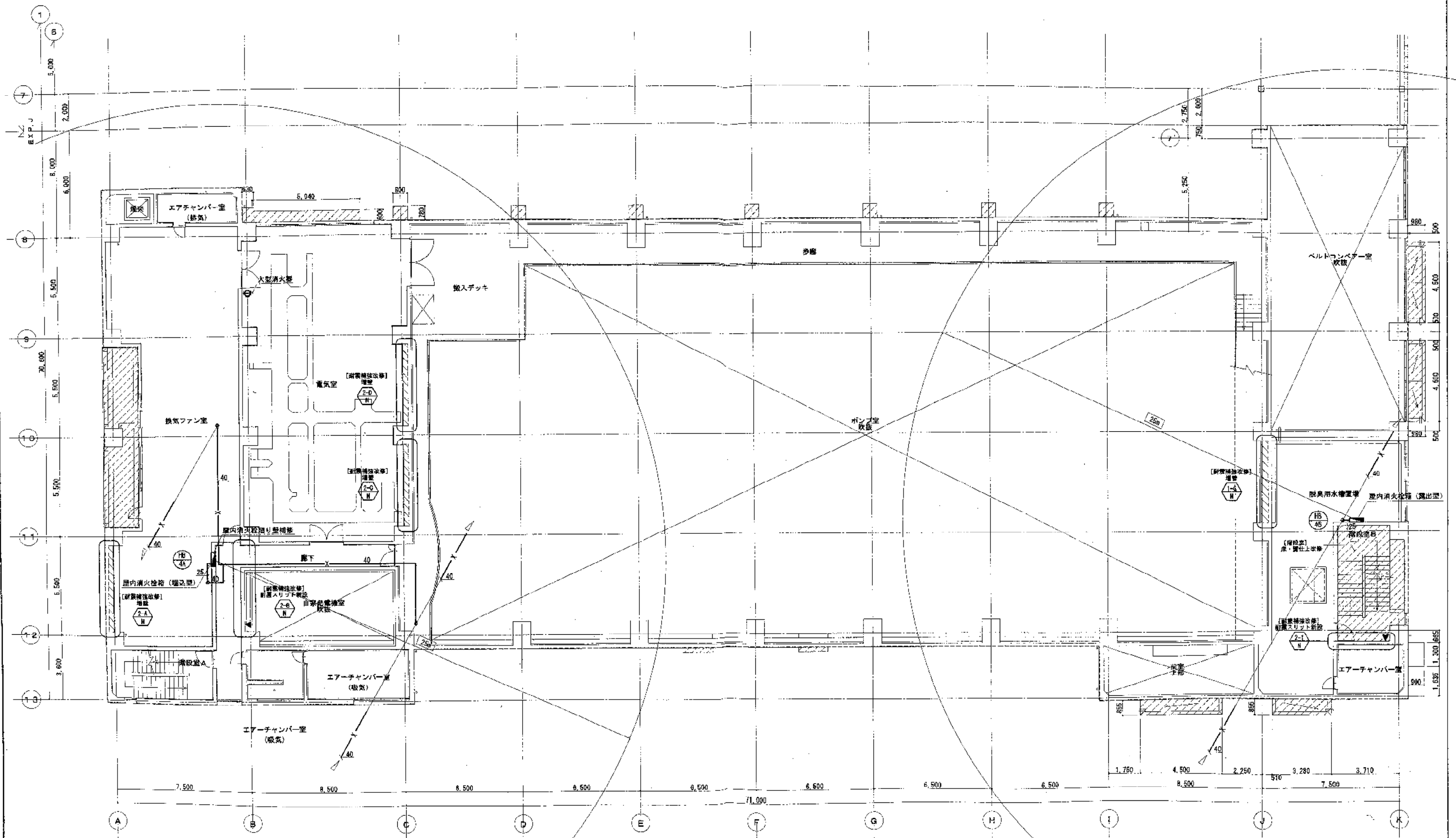
2樓 平面圖 1/100
