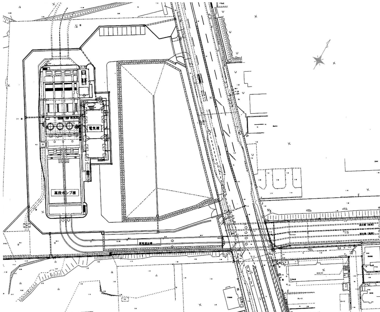
【浦安ポンプ場 一般平面図】
