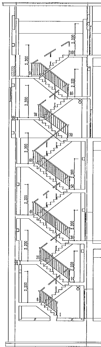
[ 階段室断面図 ]
