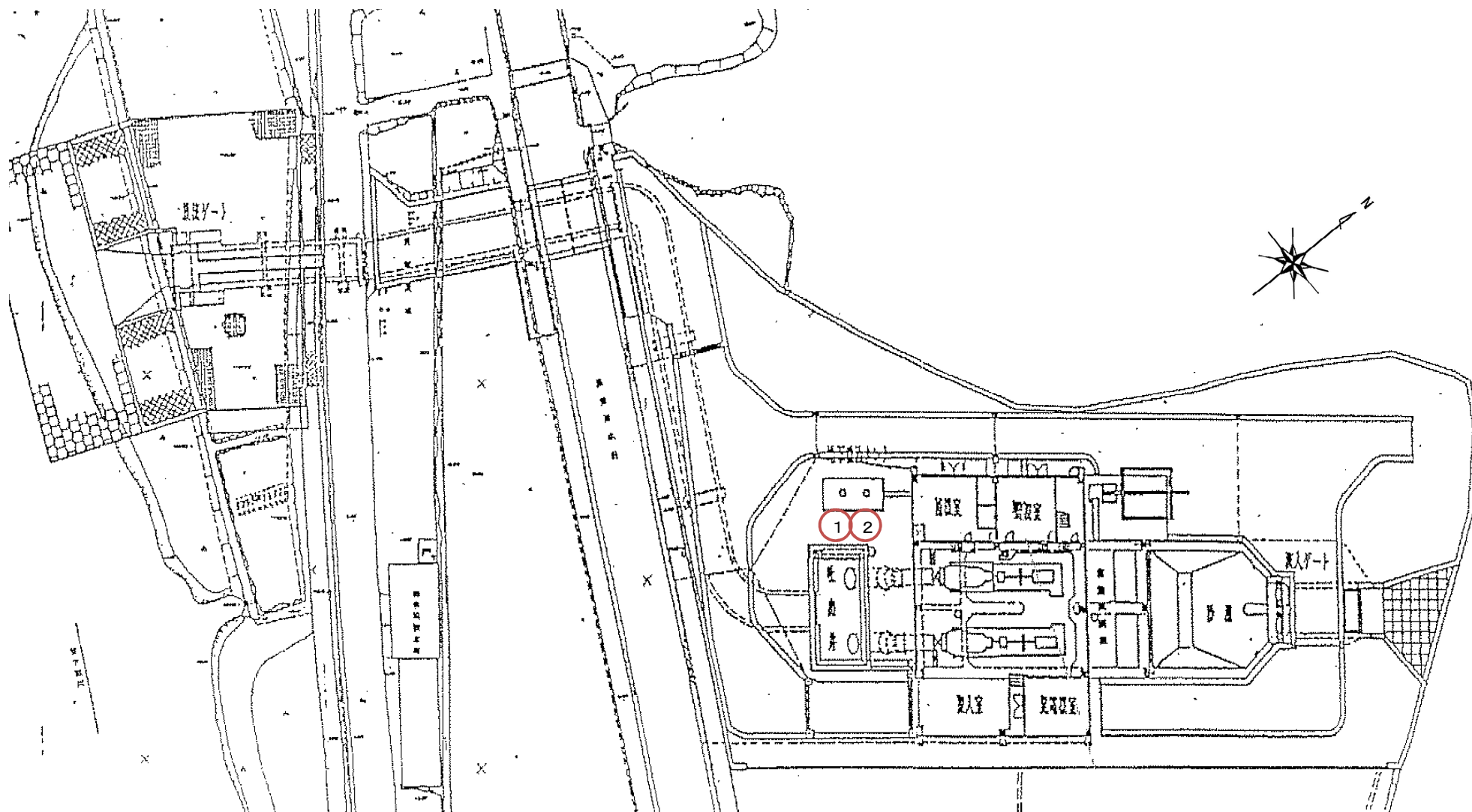
【平田ポンプ場 一般平面図】
