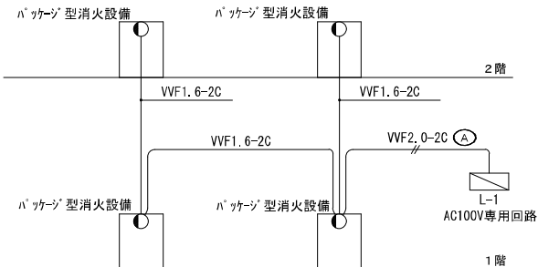
ハ「ツケ」型消火設備表示灯系統図
