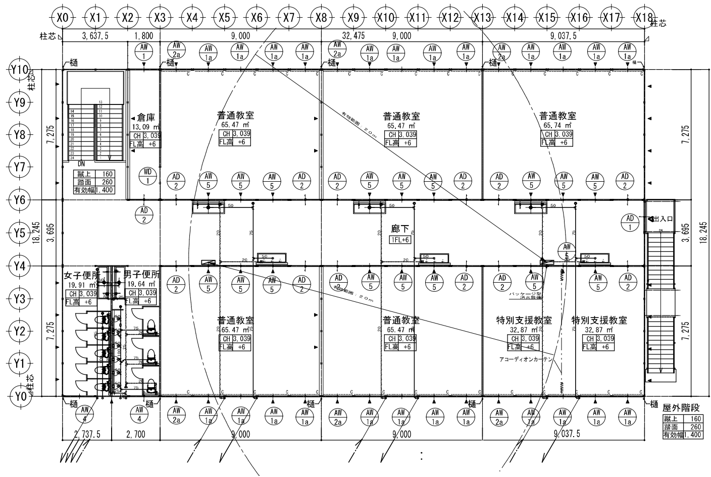
2 階平面図 S=1:100 (2階のみ：AW-5はすりガラス)
