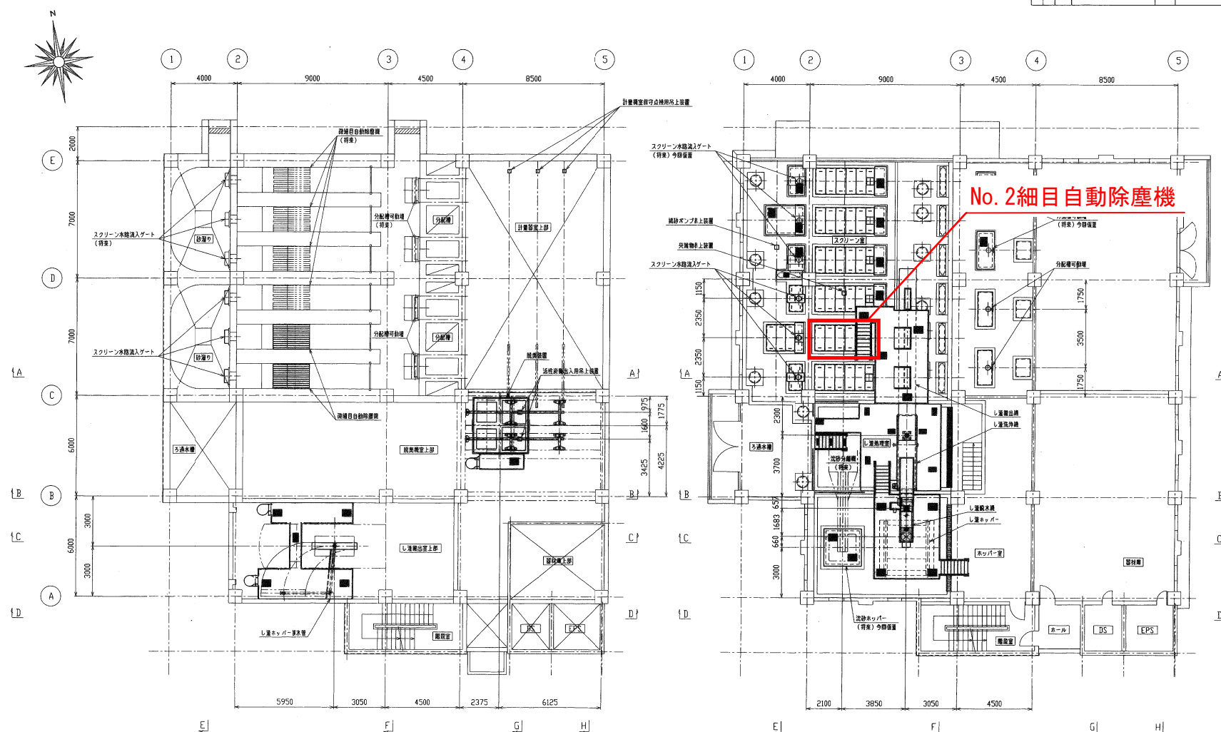
1階上部 平面図 1/100
