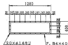
シュート開口部詳細図
