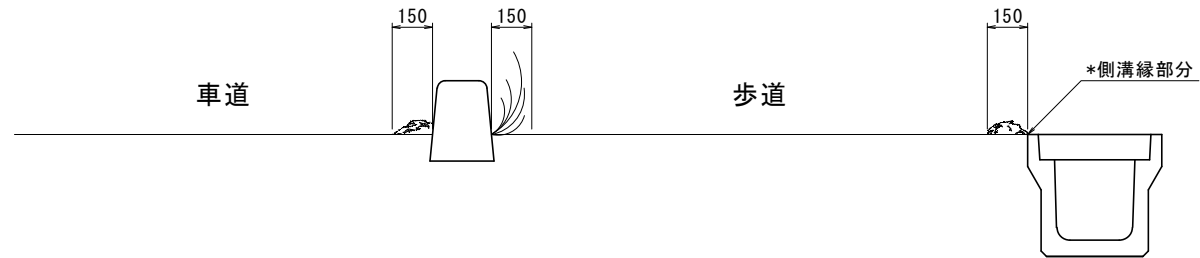
タイプ1 歩車道境界ブロック両側
