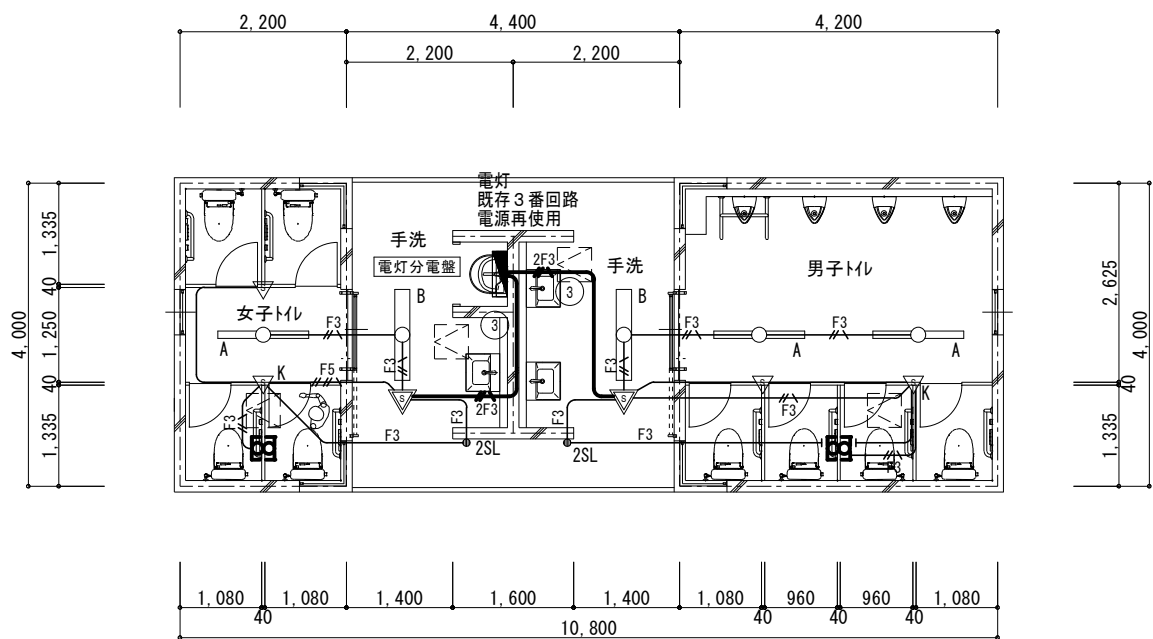
改修平面図 1:50
