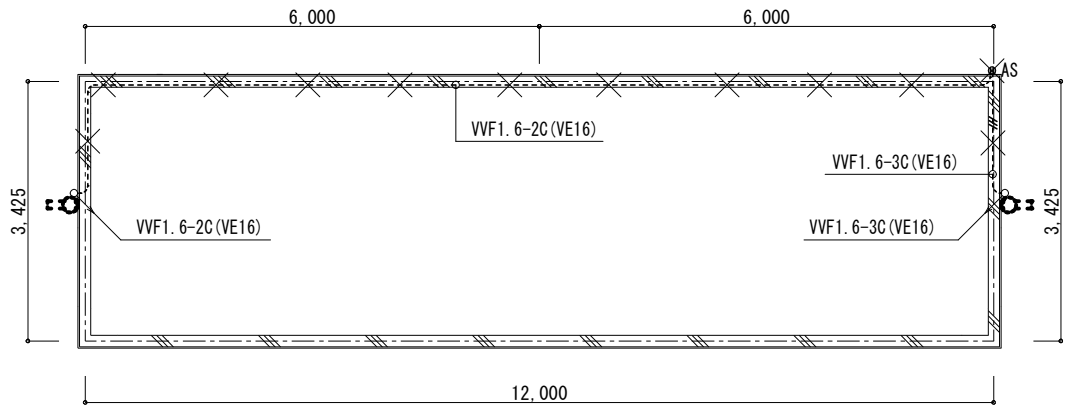
屋根伏図 1:50
