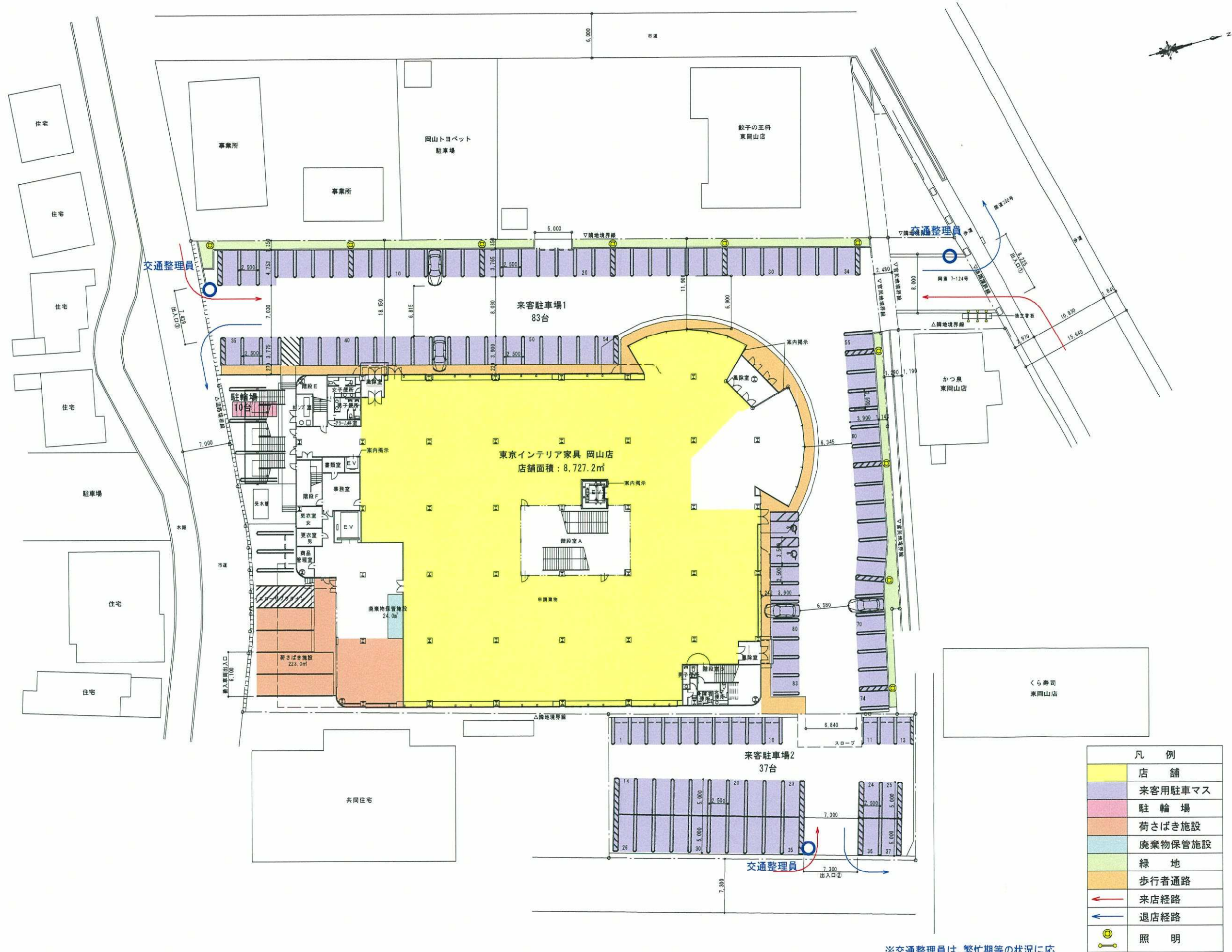
図1-3-1 建物配置図 S=1:500
