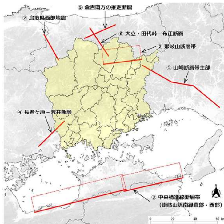
図 資 4-2 特に大きな被害をもたらすことが想定される断層型地震の断層面
