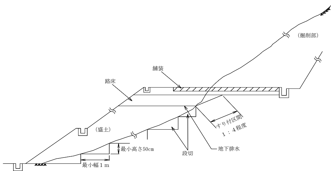
図 2 - 2 盛土基礎地盤の段切
