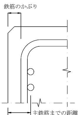
図 3 - 1 鉄筋のかぶり
